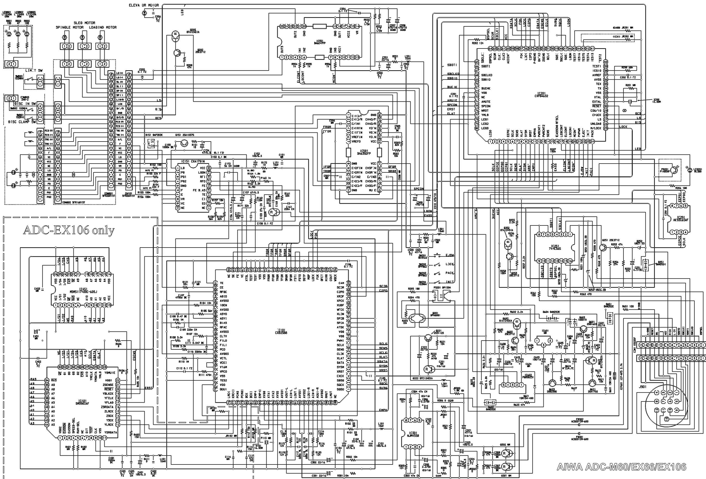
Схема автомагнитолы AIWA ADC-M60, ADC-EX66, ADC-EX106
