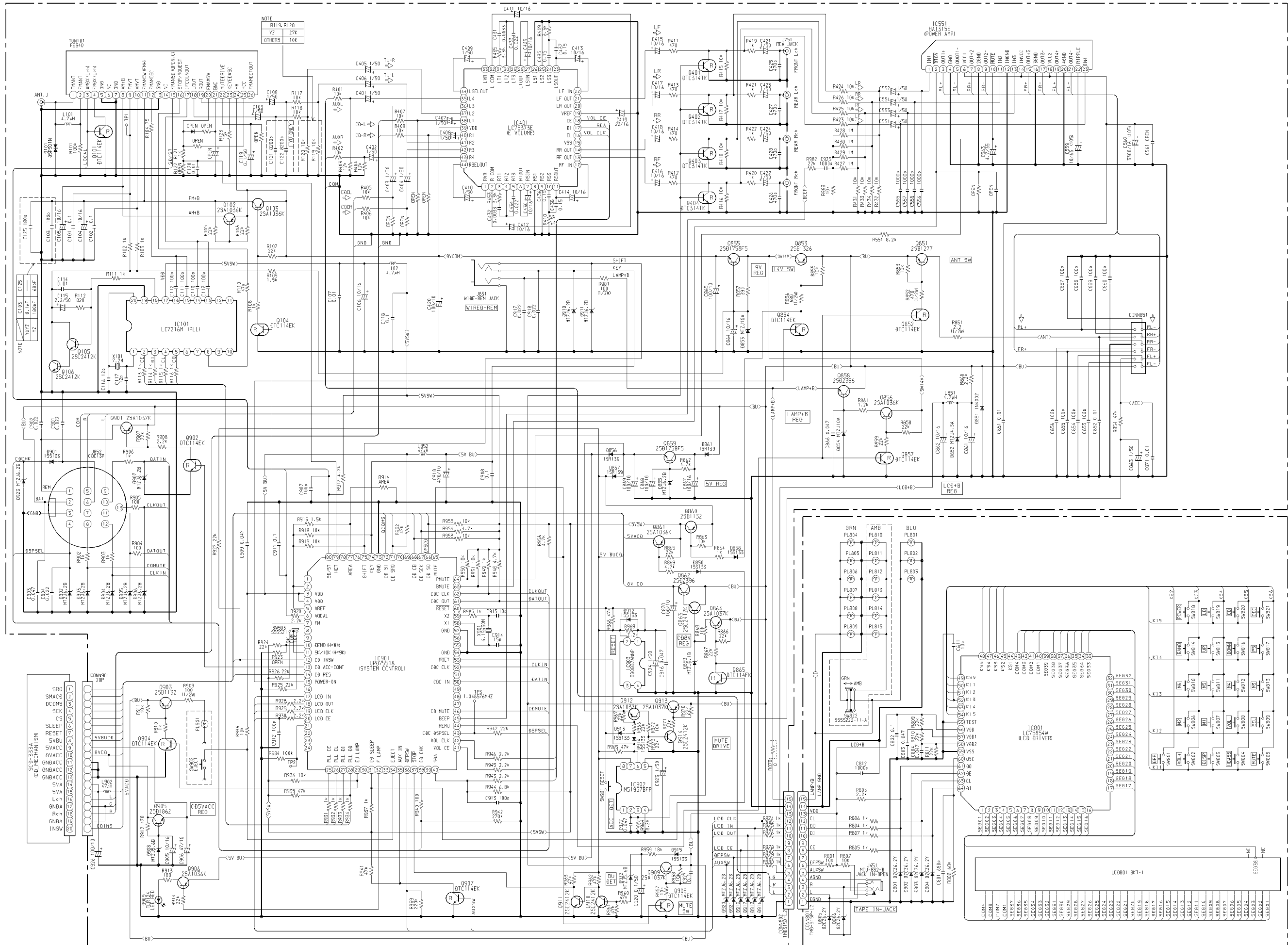
Схема автомагнитолы AIWA CDC-X175
