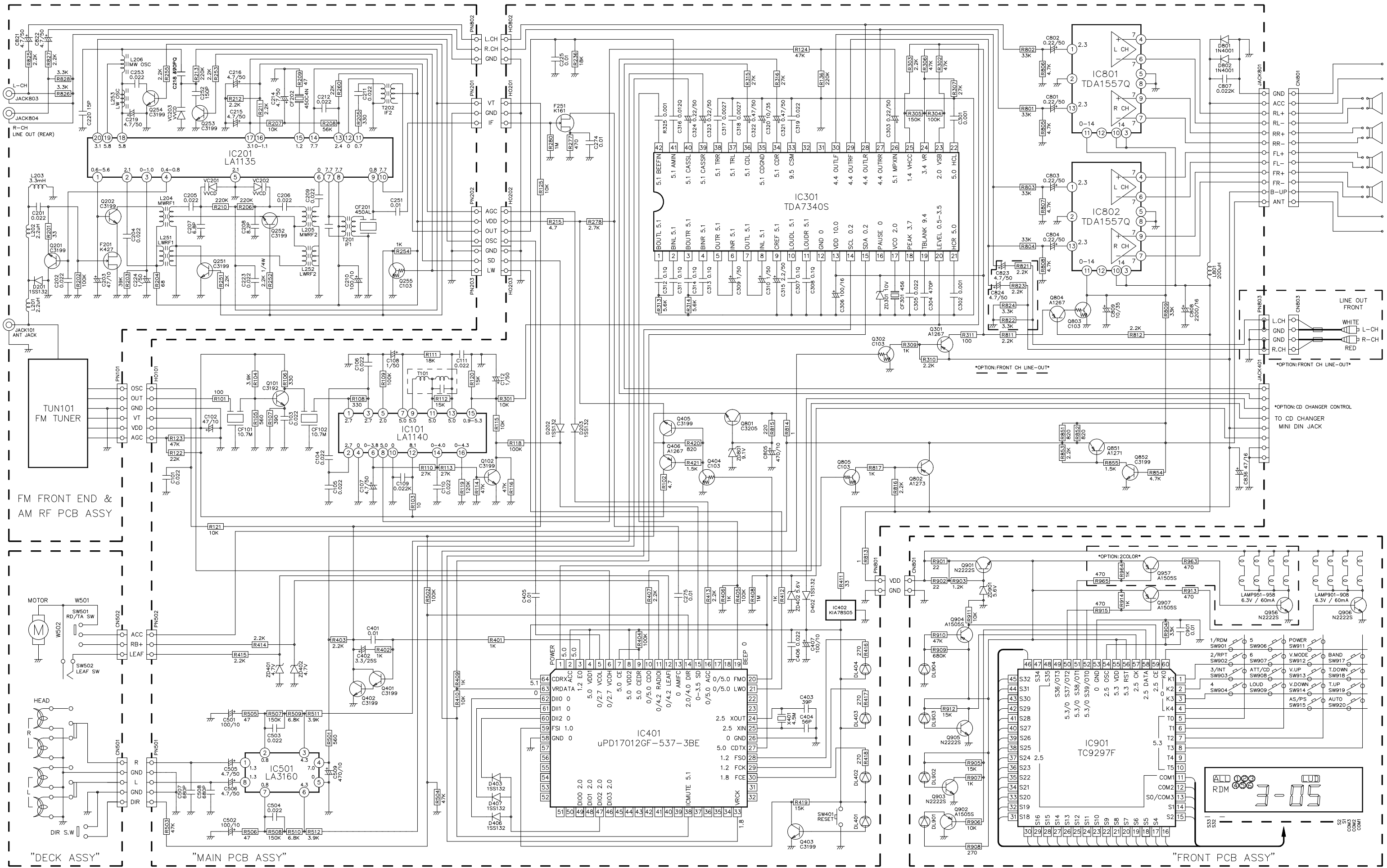
Схема автомагнитолы LG 570/670
