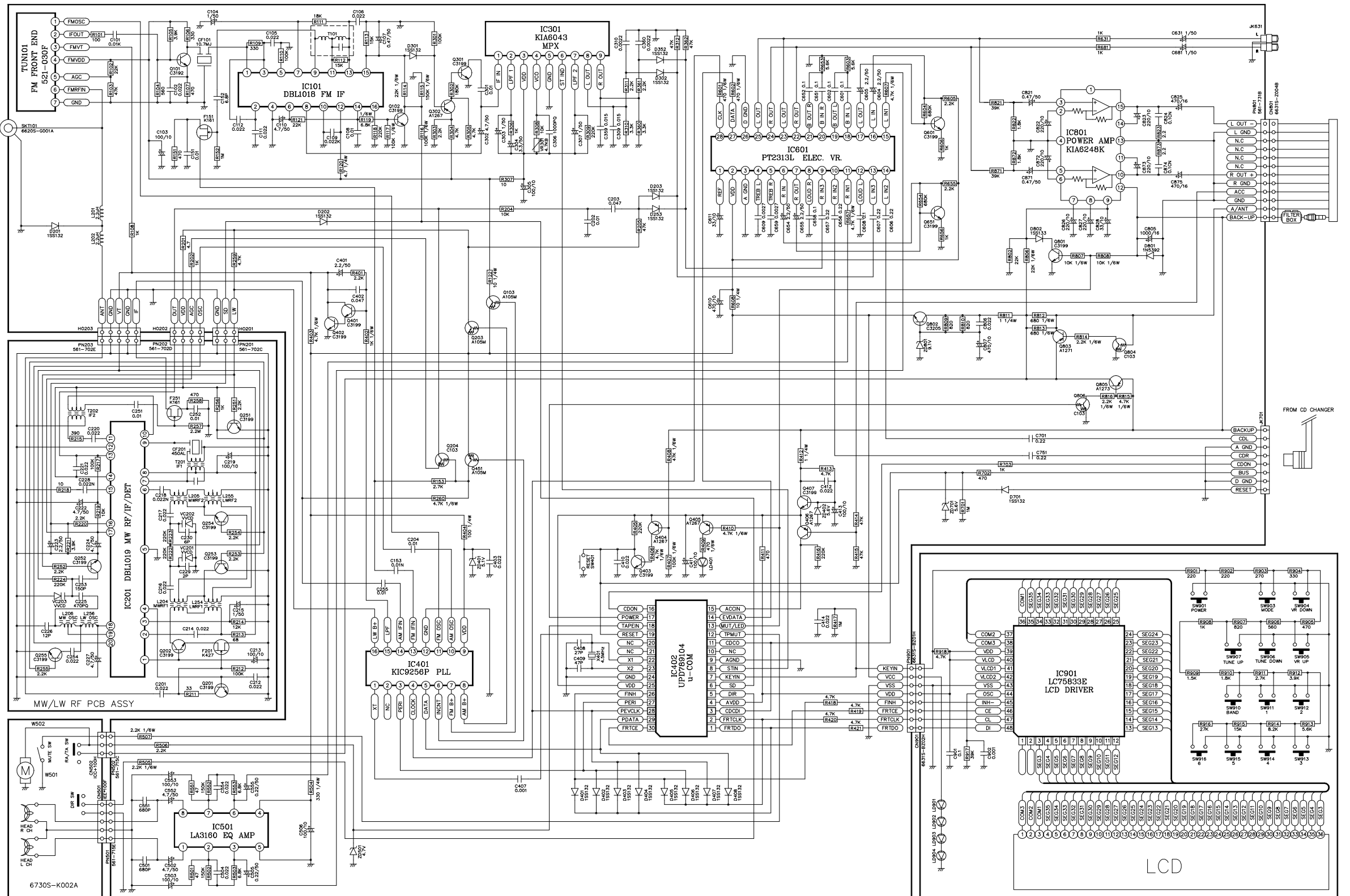
Схема автомагнитолы LG TCC2010
