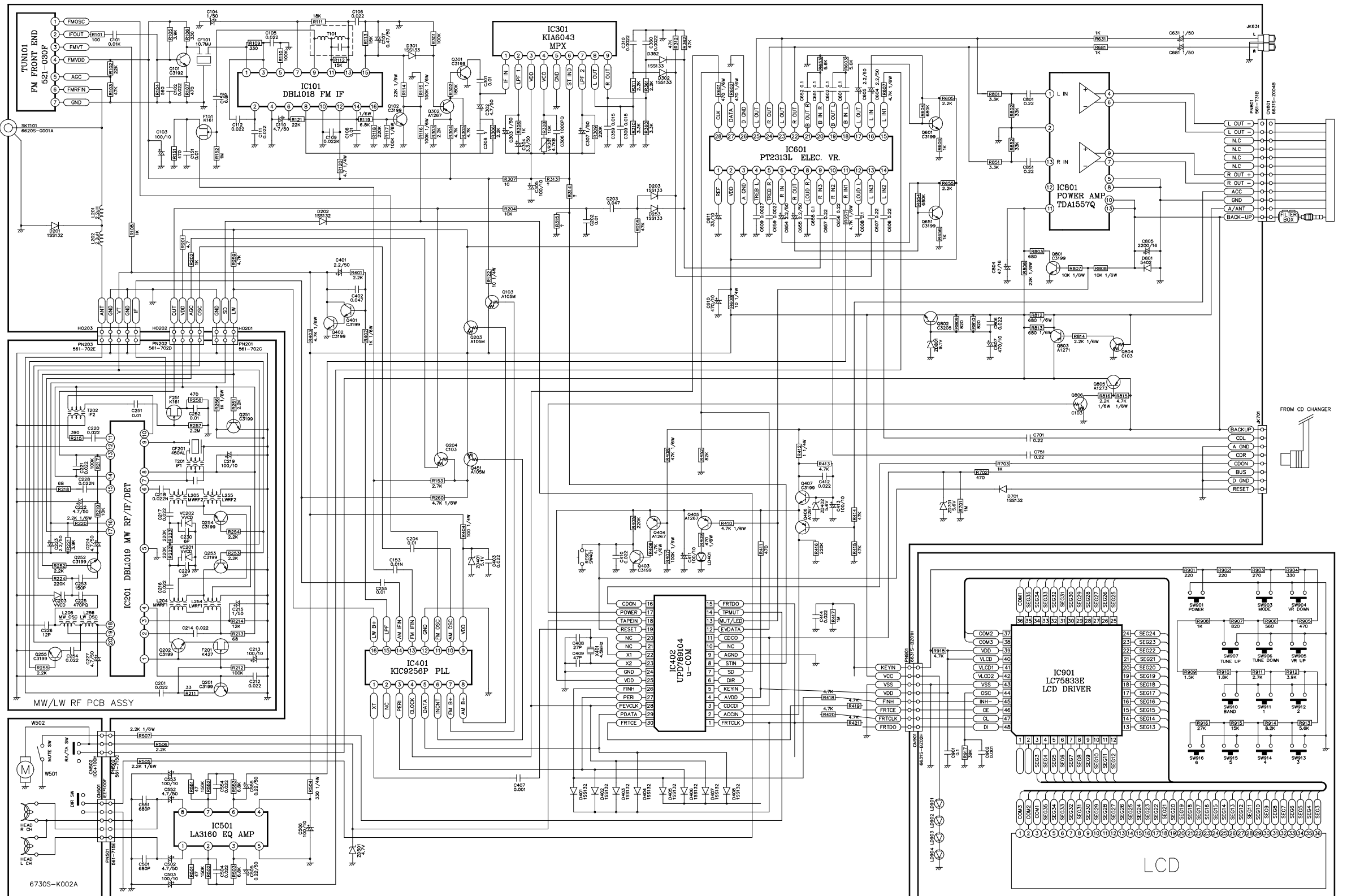
Схема автомагнитолы LG TCC2510, TCC2515
