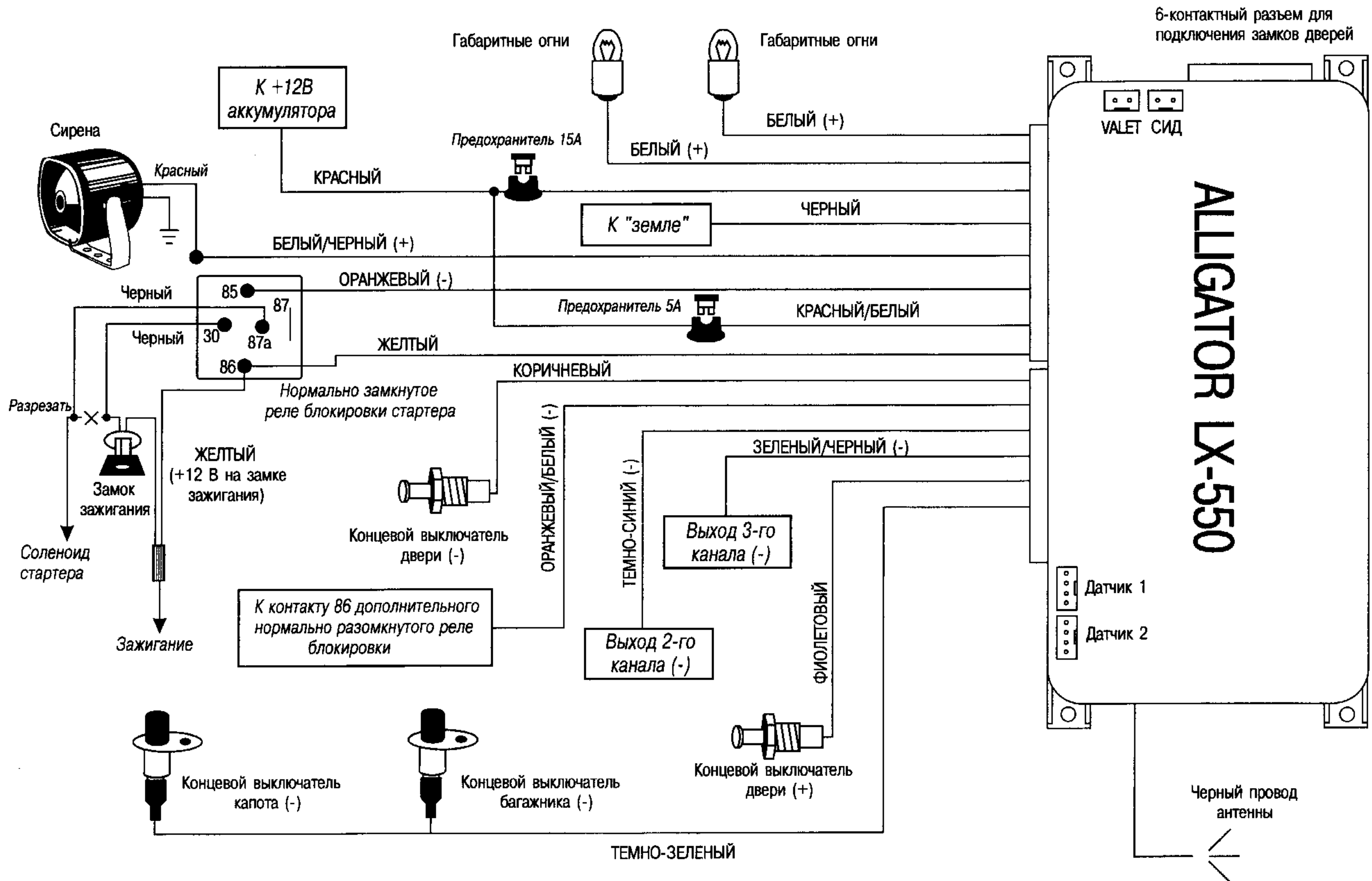
Схема подключения автосигнализации Alligator LX-550
