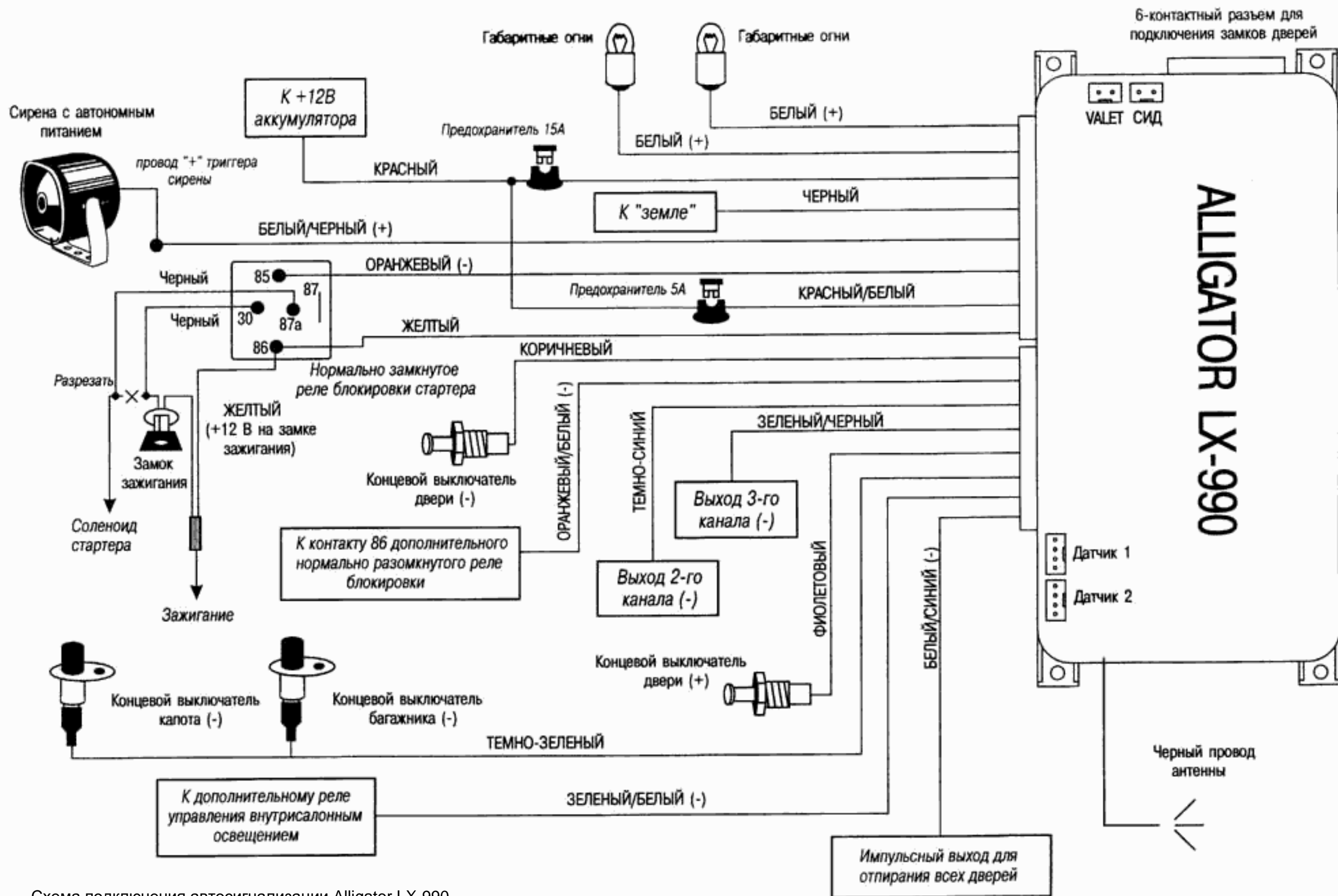
Схема подключения автосигнализации Alligator LX-990
