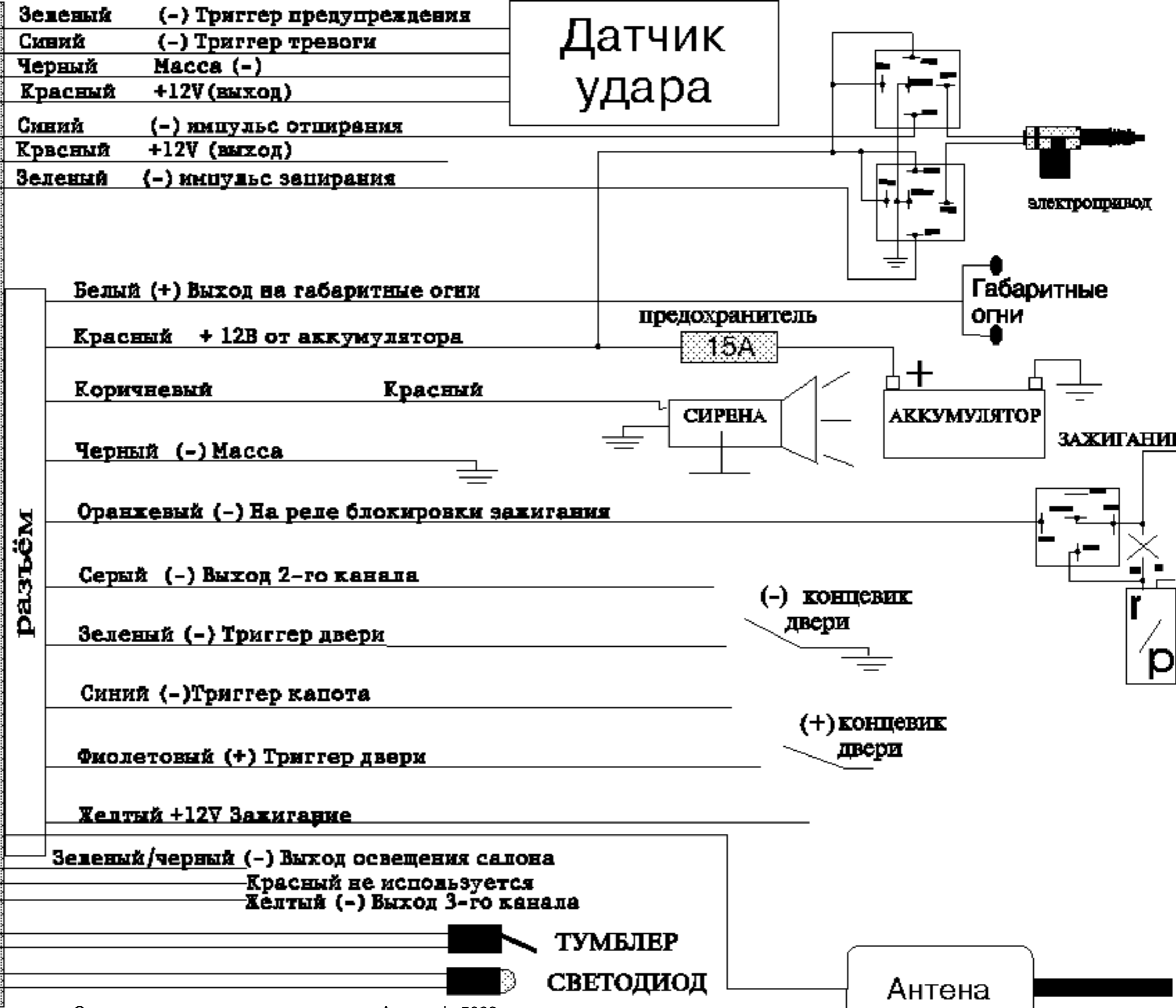
Схема подключения автосигнализации Anaconda 5000
