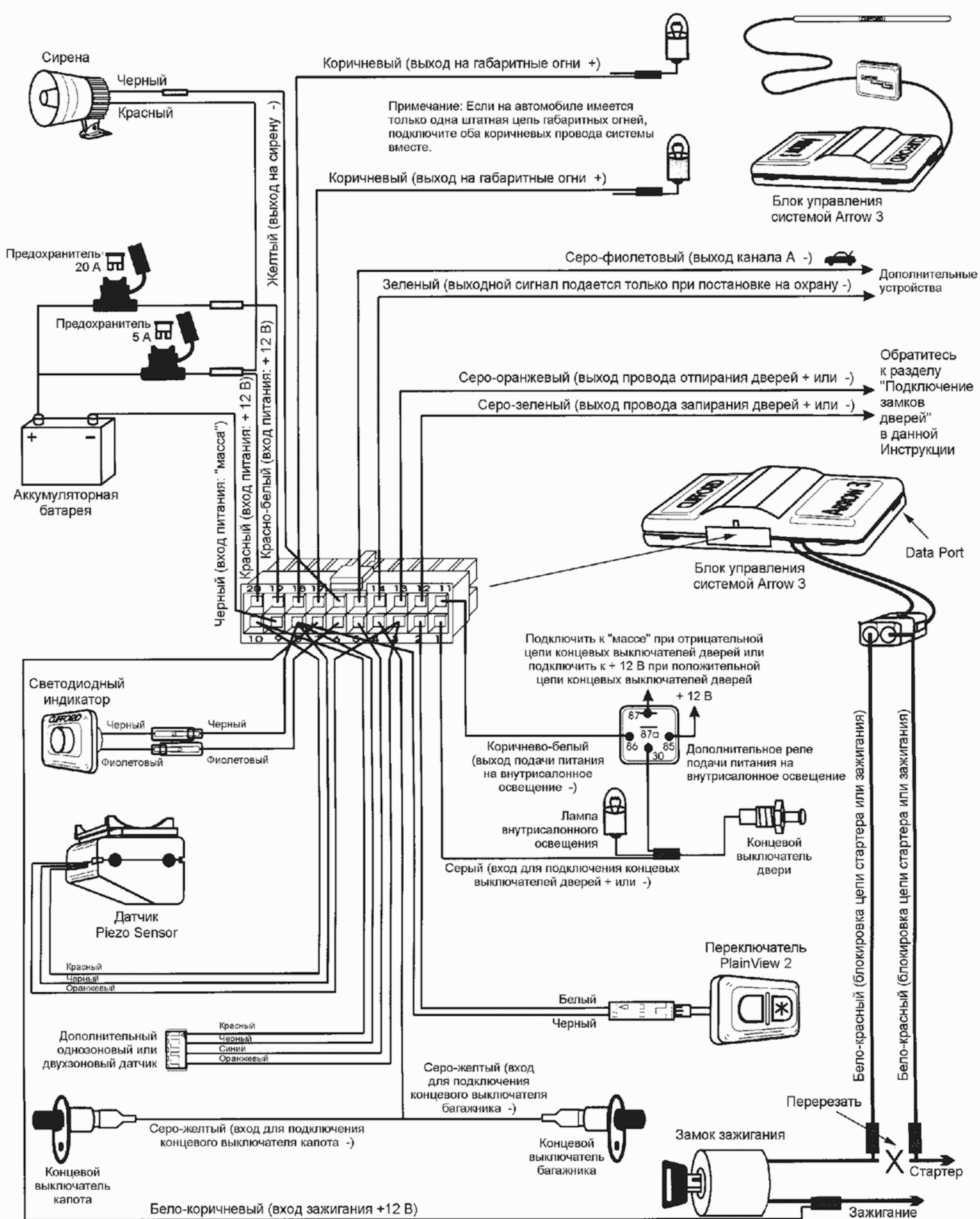
Схема подключения автосигнализации Clifford Arrow 3
