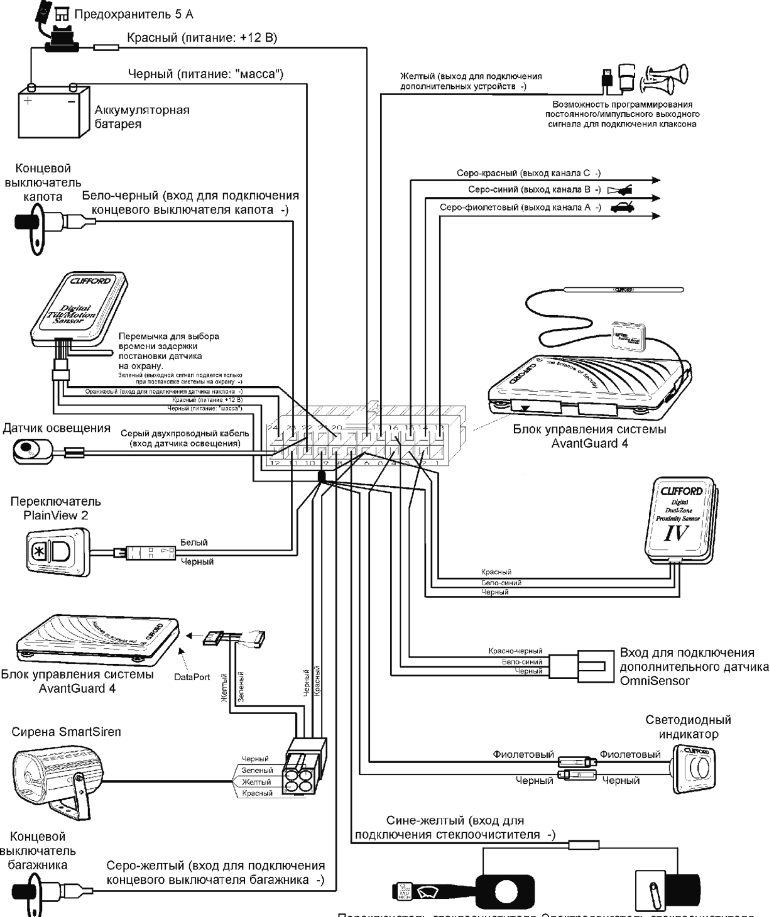
Схема подключения автосигнализации Clifford AvantGuard 4
