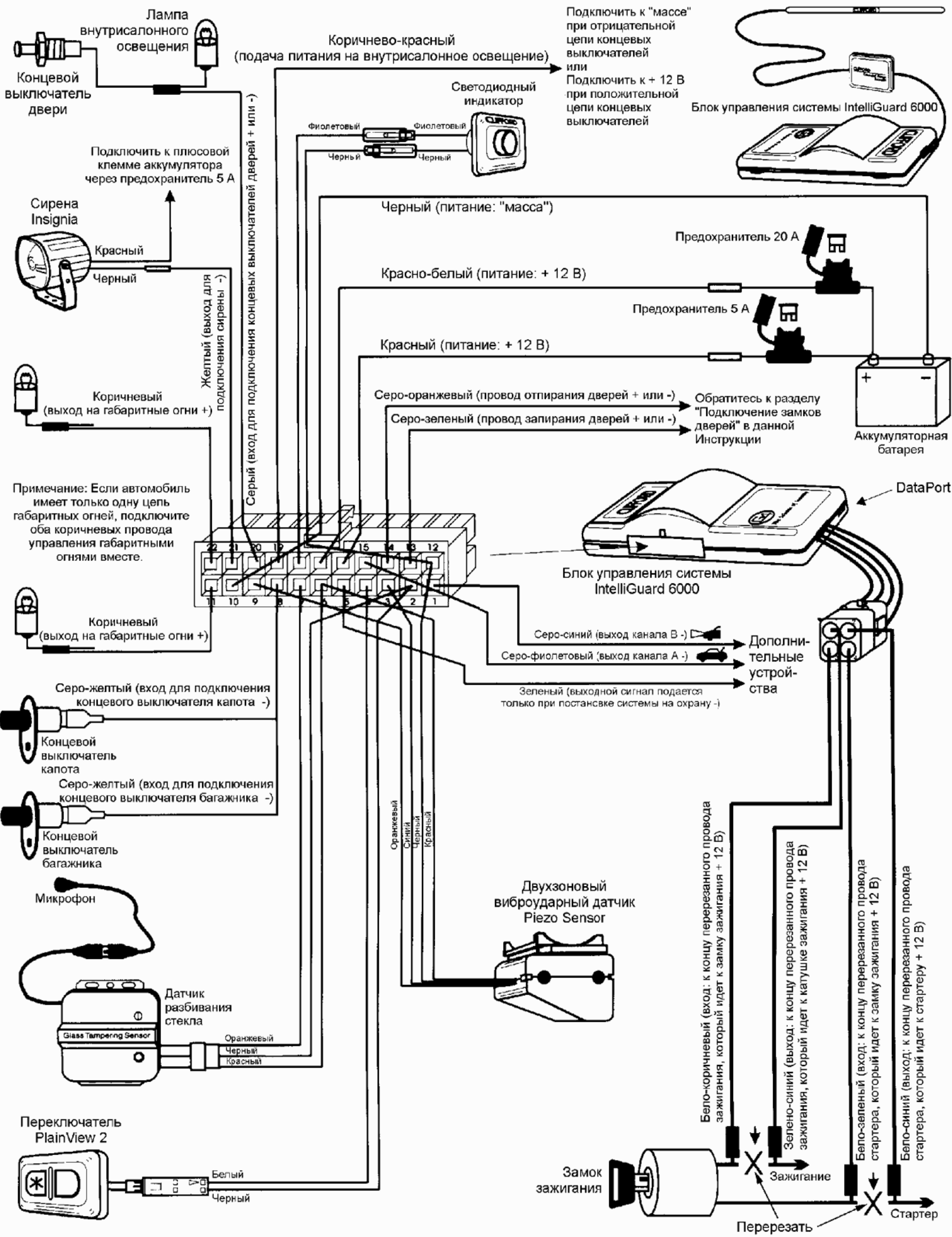
Схема подключения автосигнализации Clifford IntelliGuard 6000
