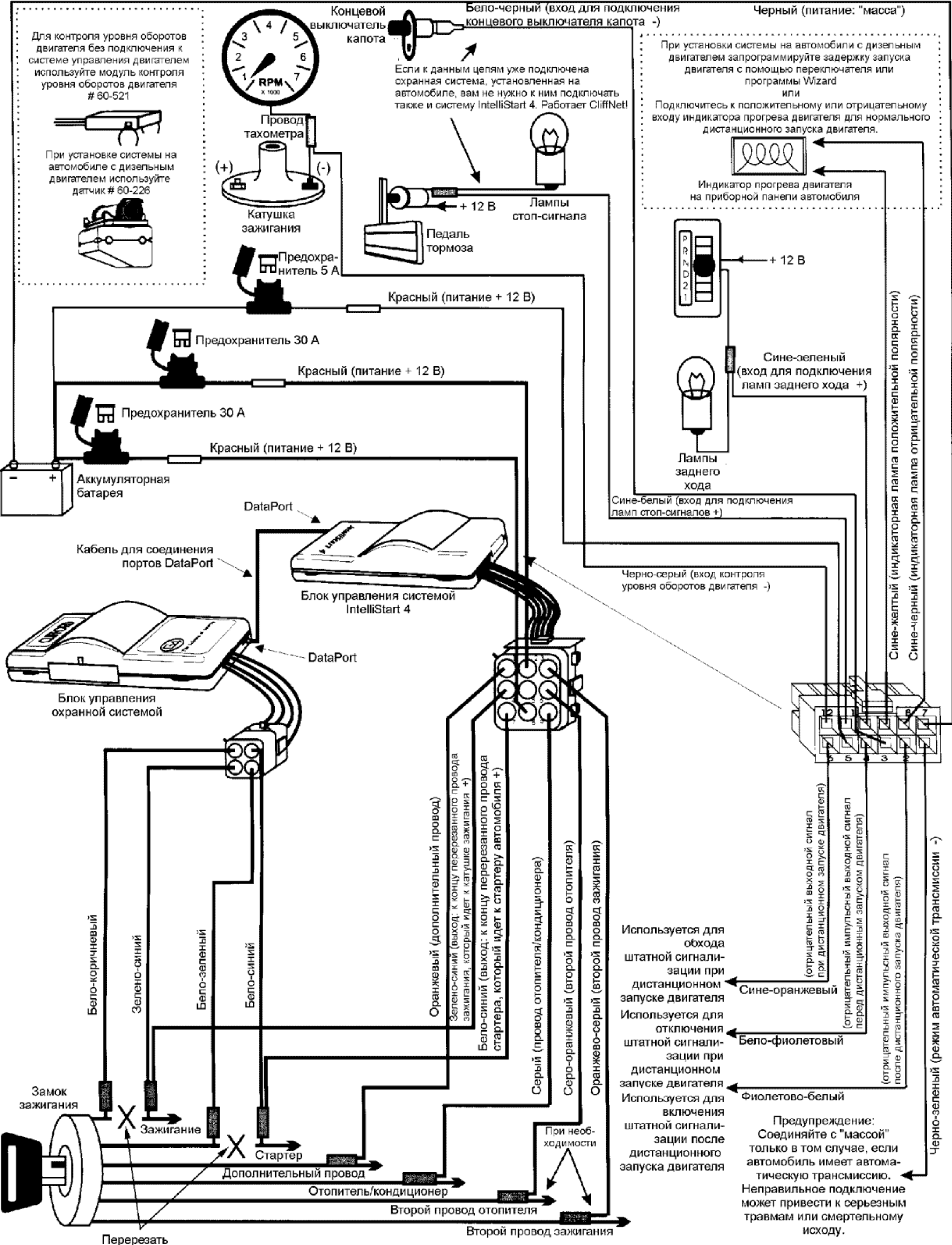
Схема подключения автосигнализации Clifford IntelliStart 4
