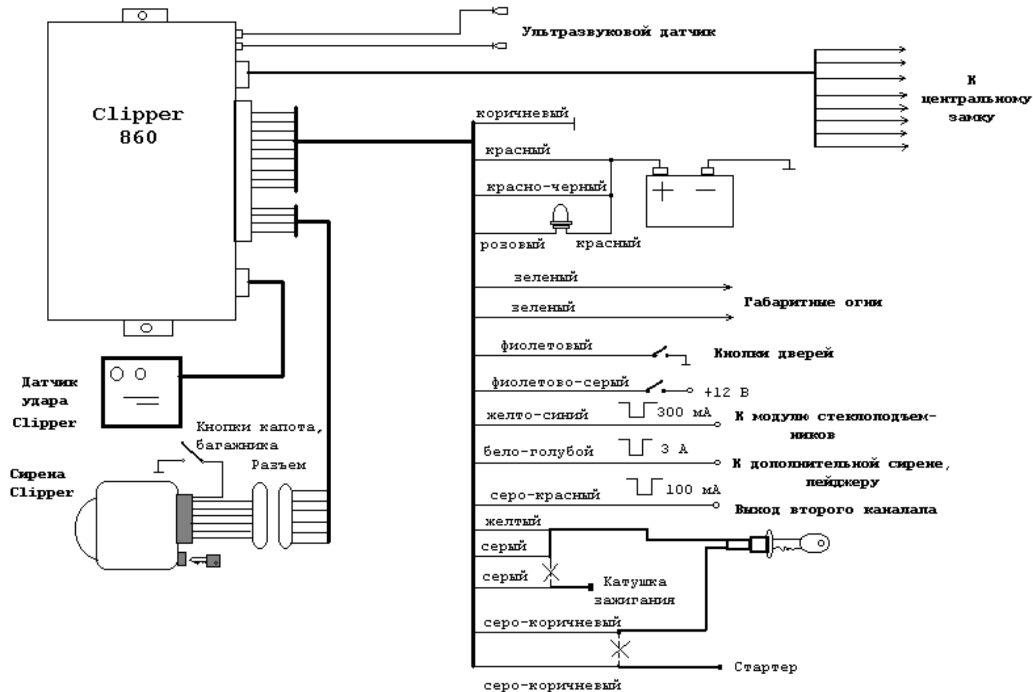
Схема подключения автосигнализации Clipper 860
