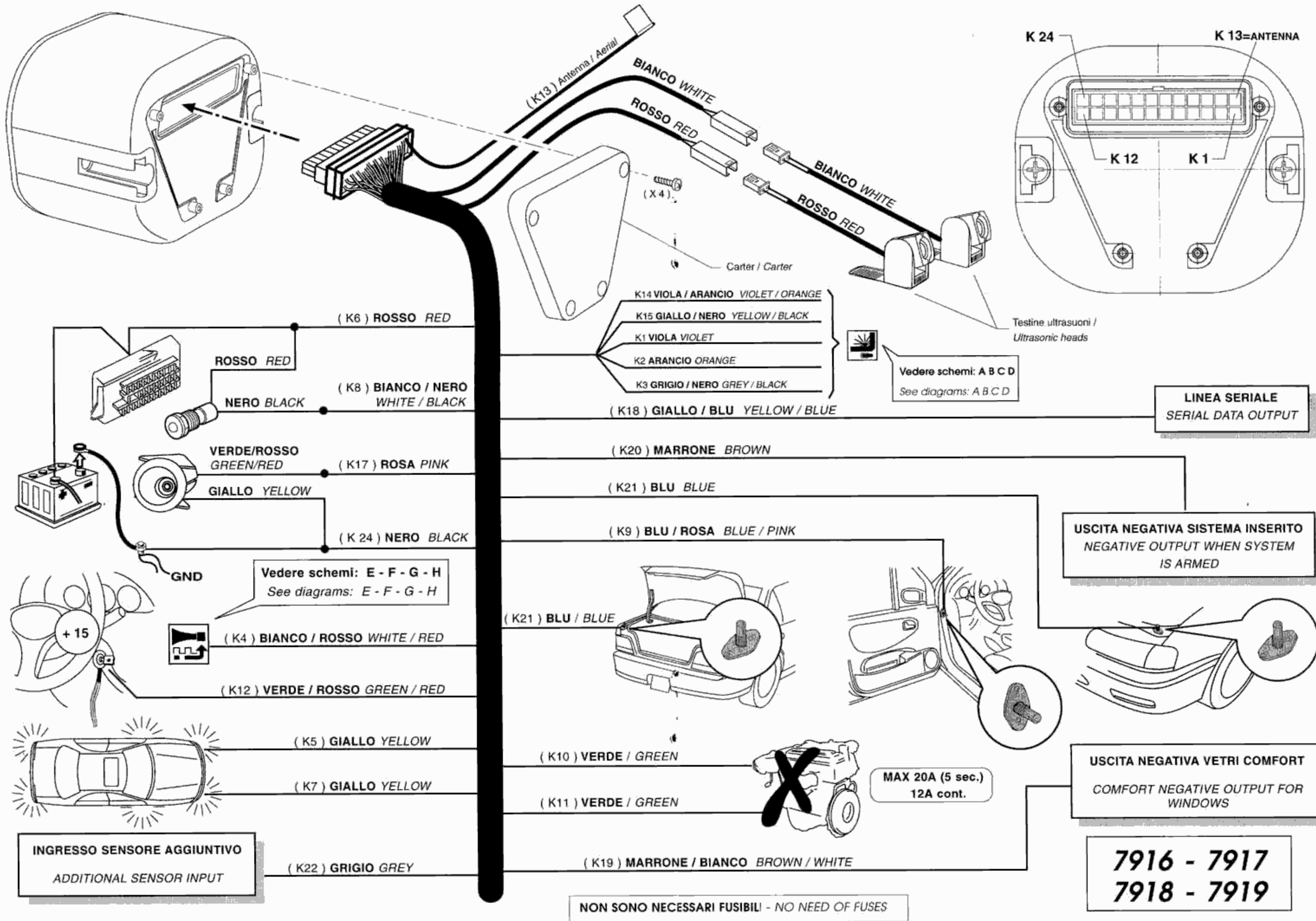
Схема подключения автосигнализации Cobra 7916/ 7917/ 7918/ 7919
