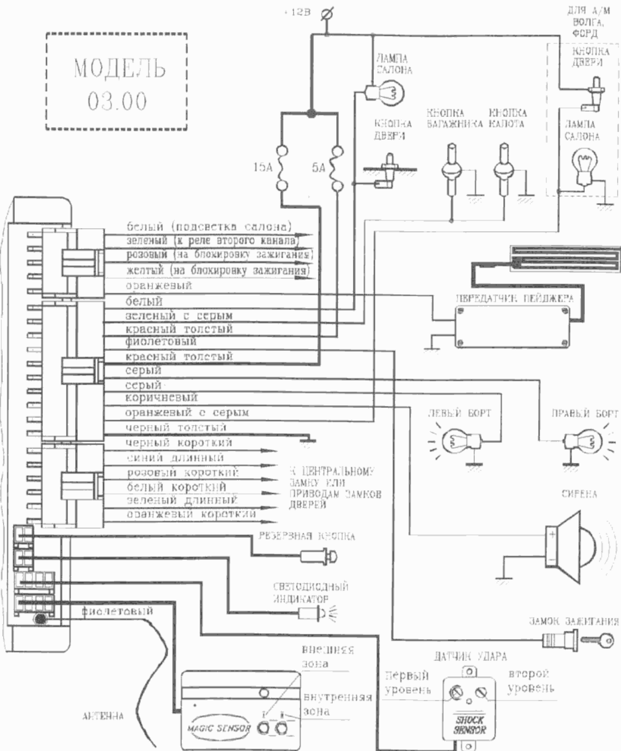
Схема подключения автосигнализации Excellent
