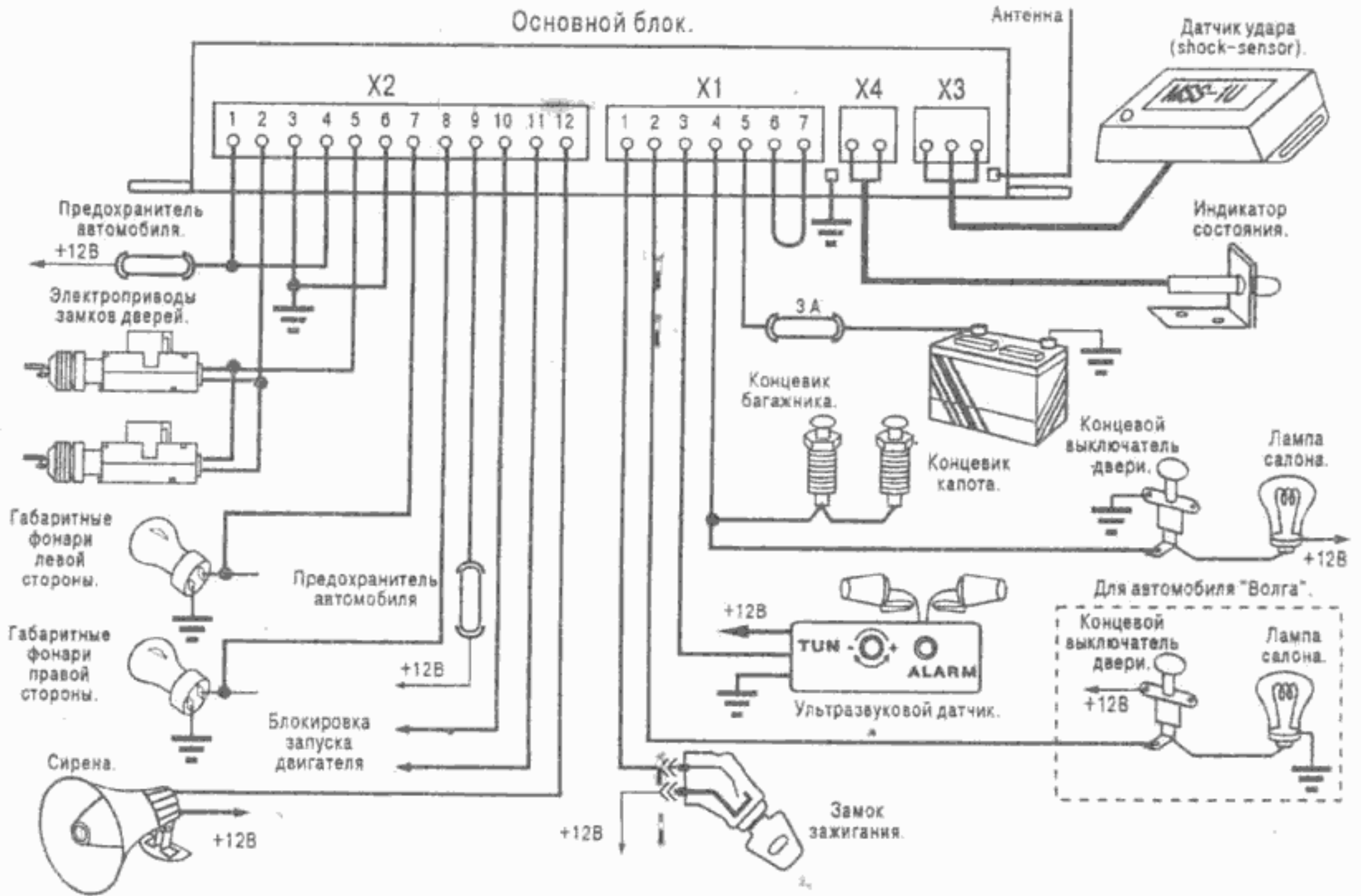
Схема основных подключений RF-100.
