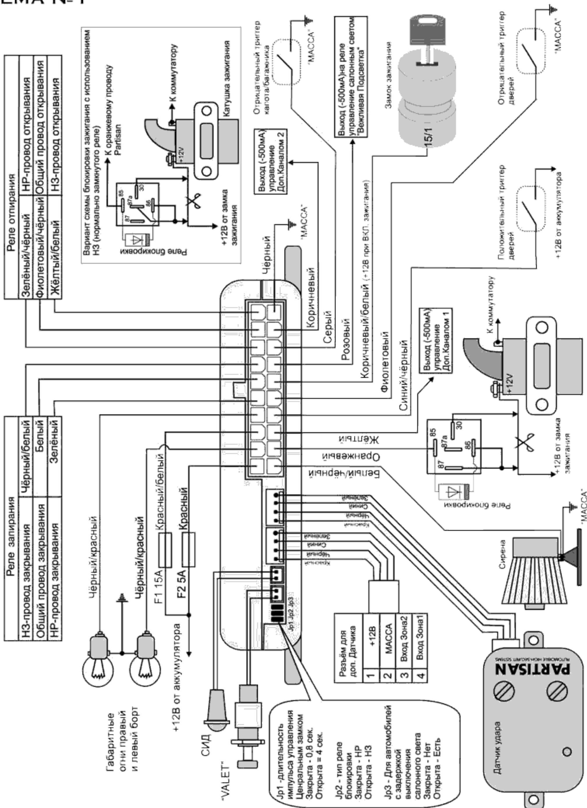
Схема подключения системы PARTISAN RX-3
