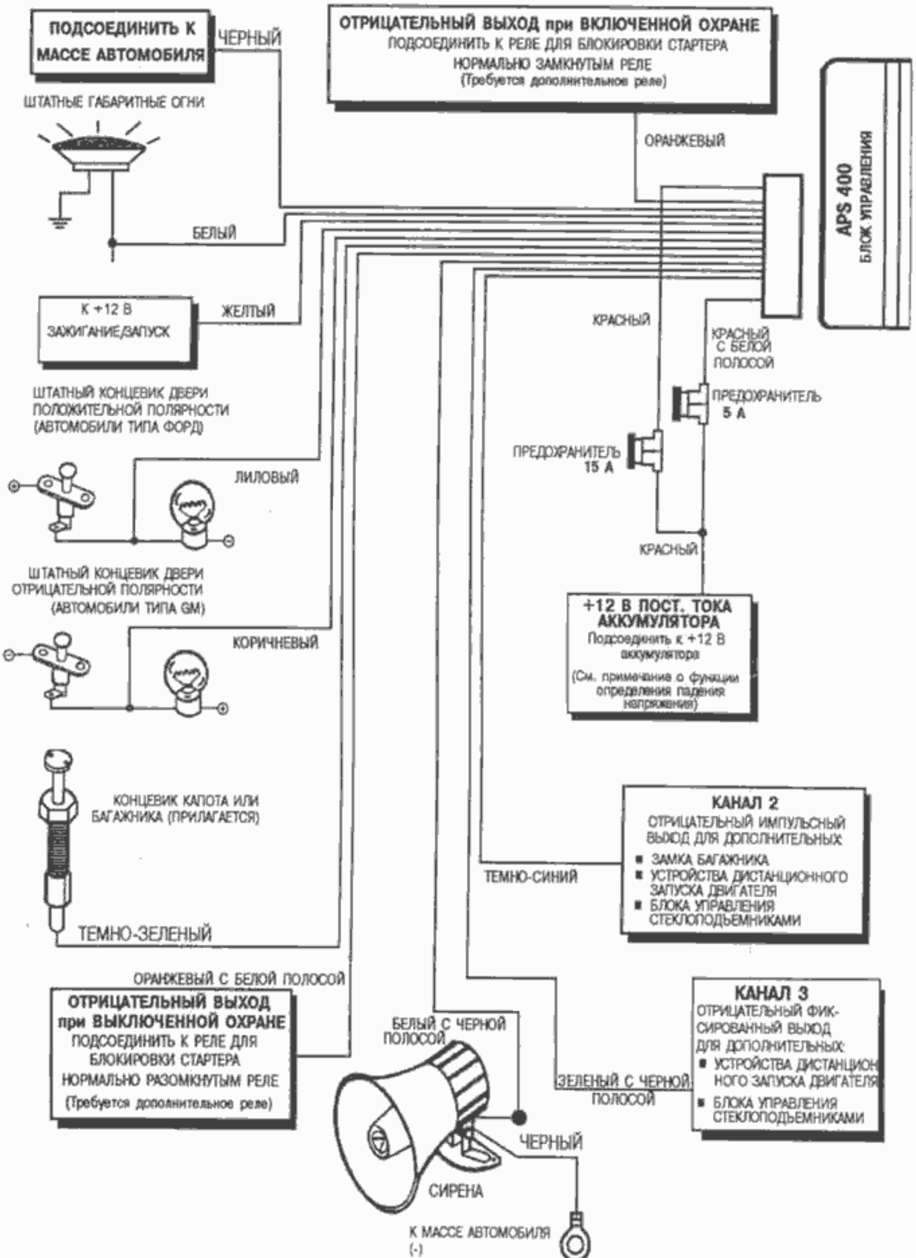
Схема подключения автосигнализации Prestige APS-400
