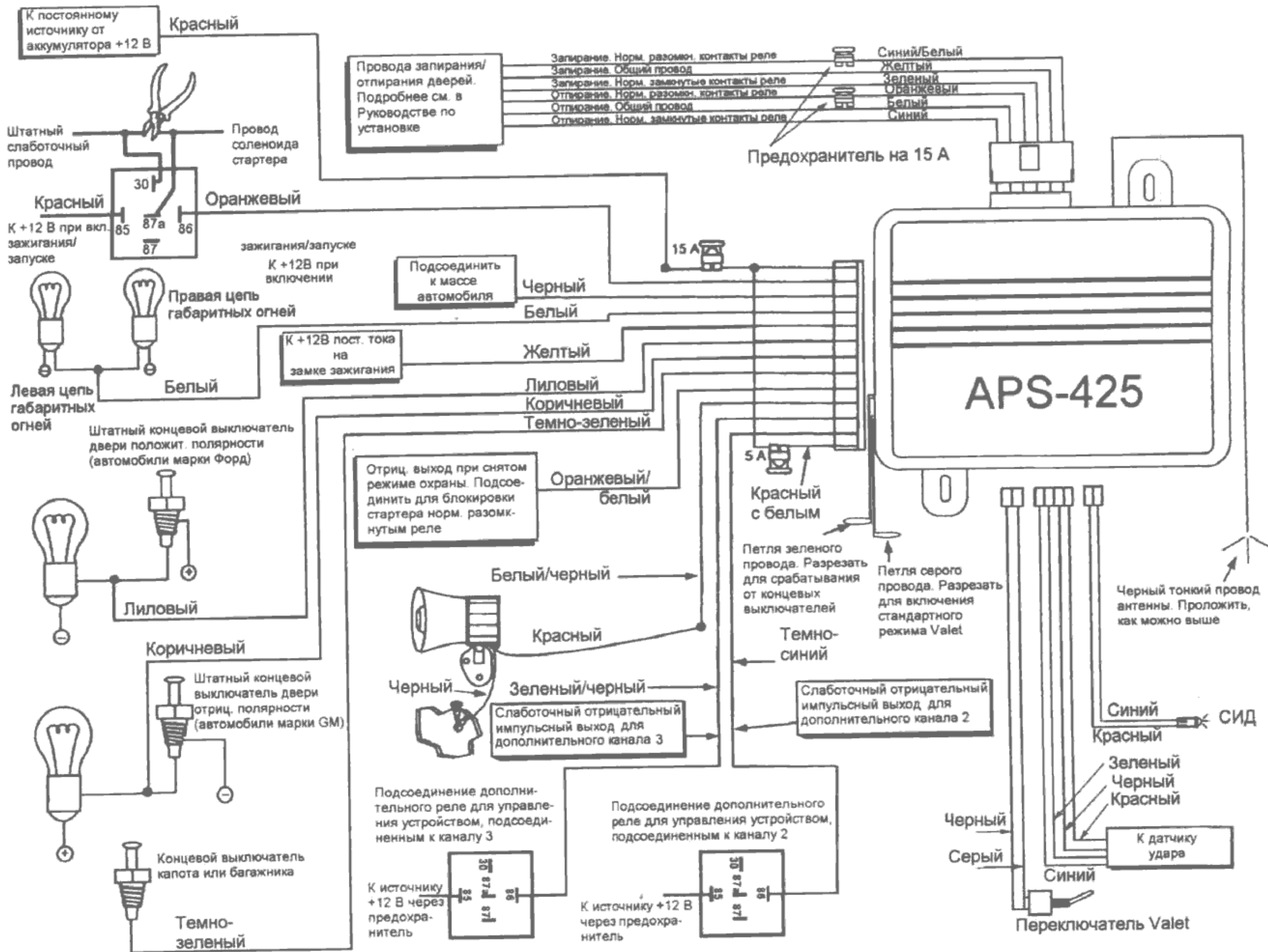
Схема подключения автосигнализации Prestige APS-425
