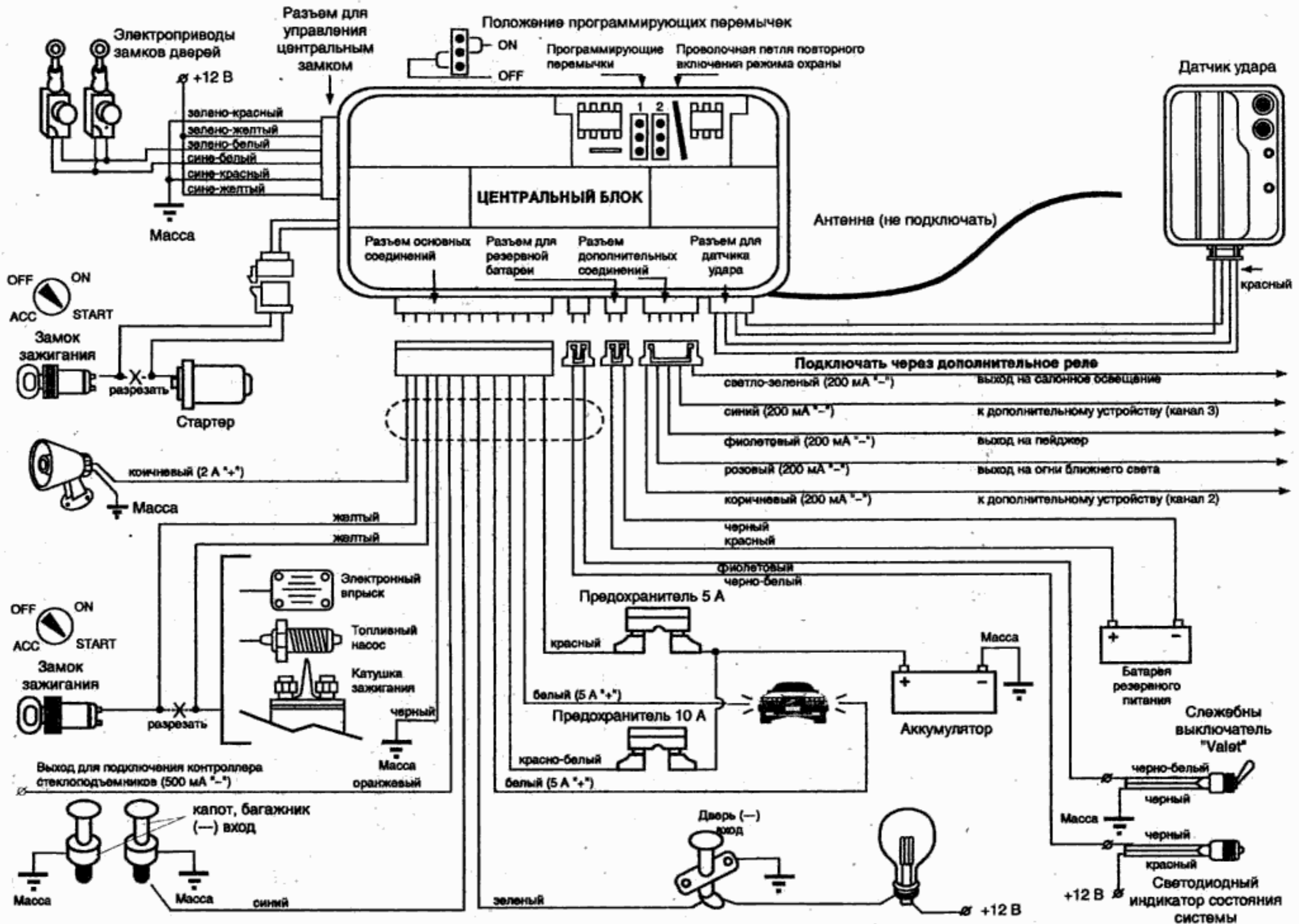
Схема подключения автосигнализации Red Scorpio SRS-2000
