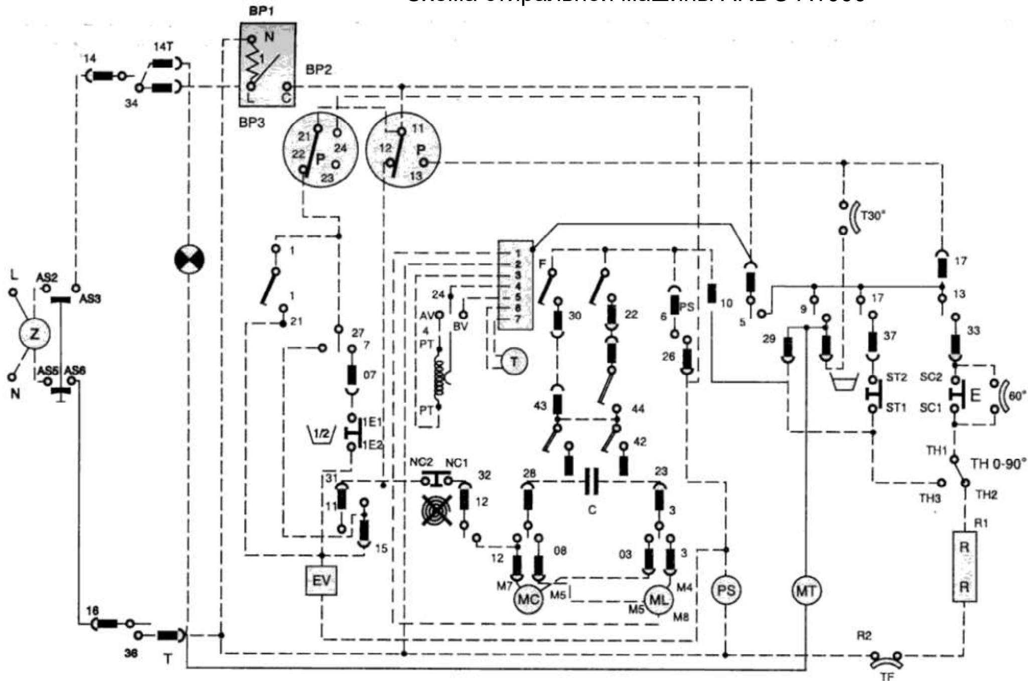
Электрическая схема стиральной машины ARDO A1000
