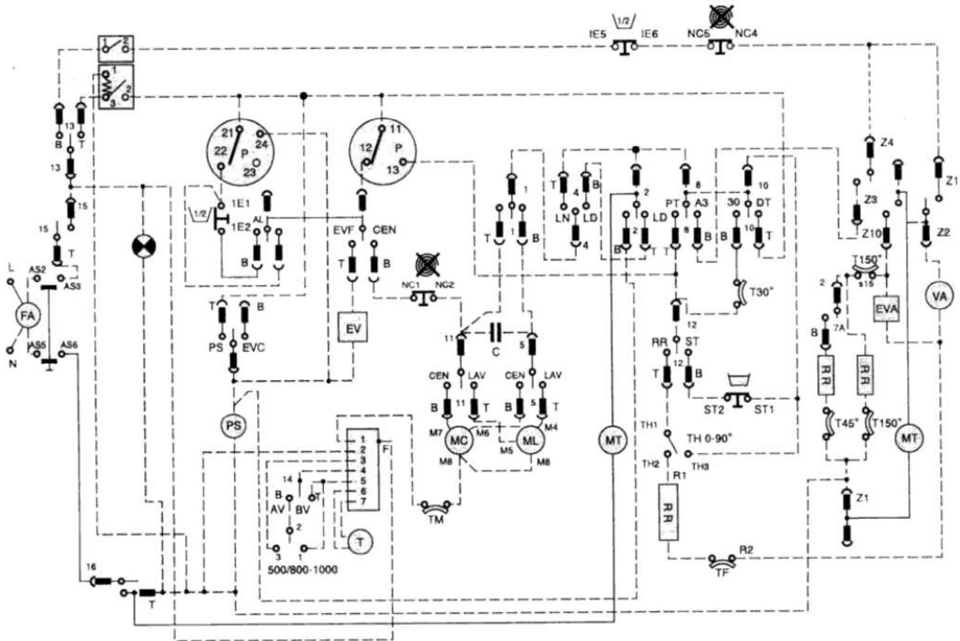
Электрическая схема стиральной машины ARDO WD800
