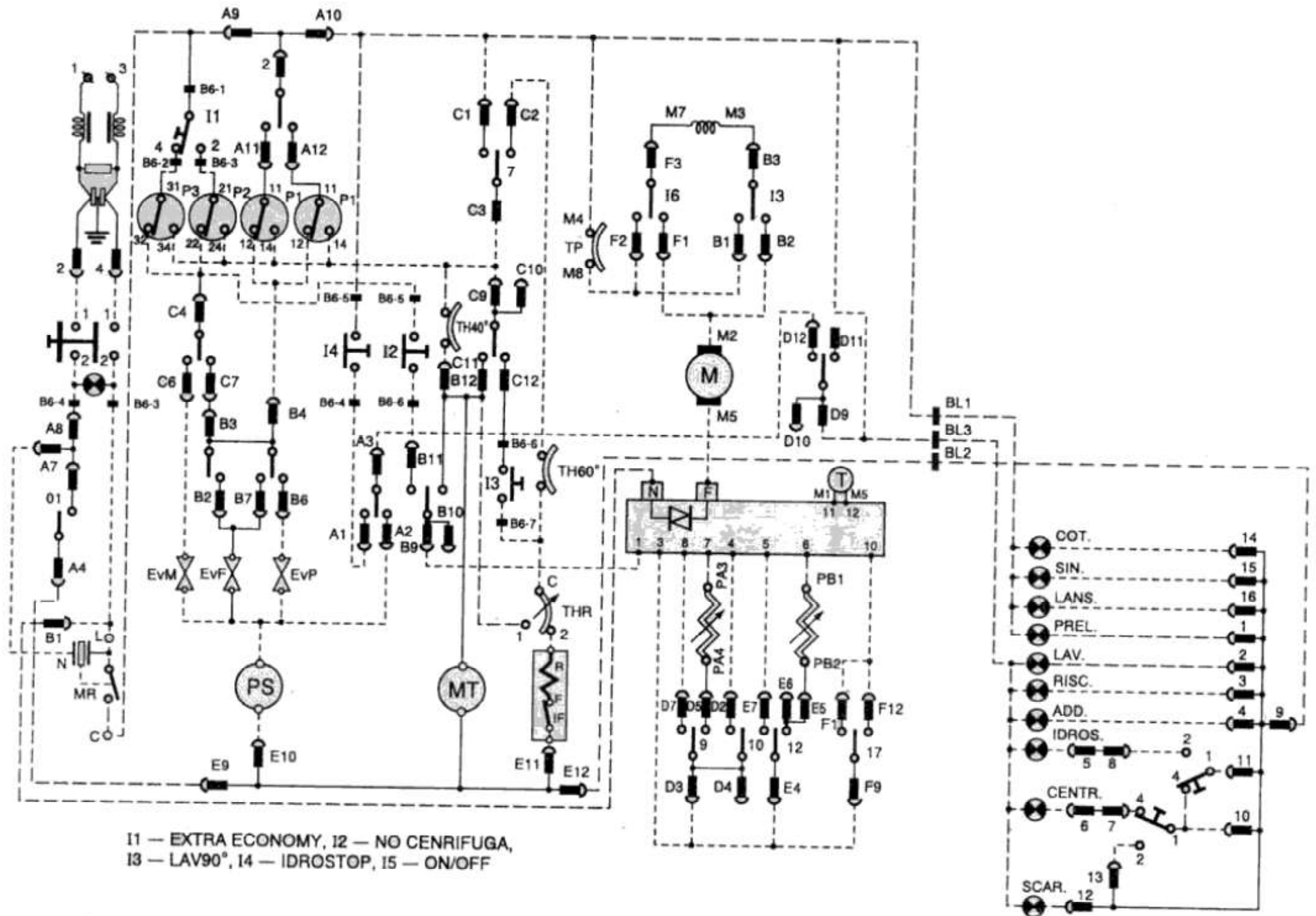
Электрическая схема стиральной машины ARISTON AM1274XRF
