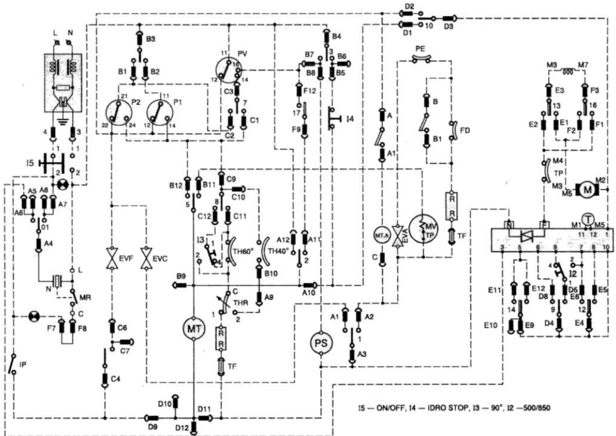
Электрическая схема стирально-сушильной машины ARISTON K-CD12TX
