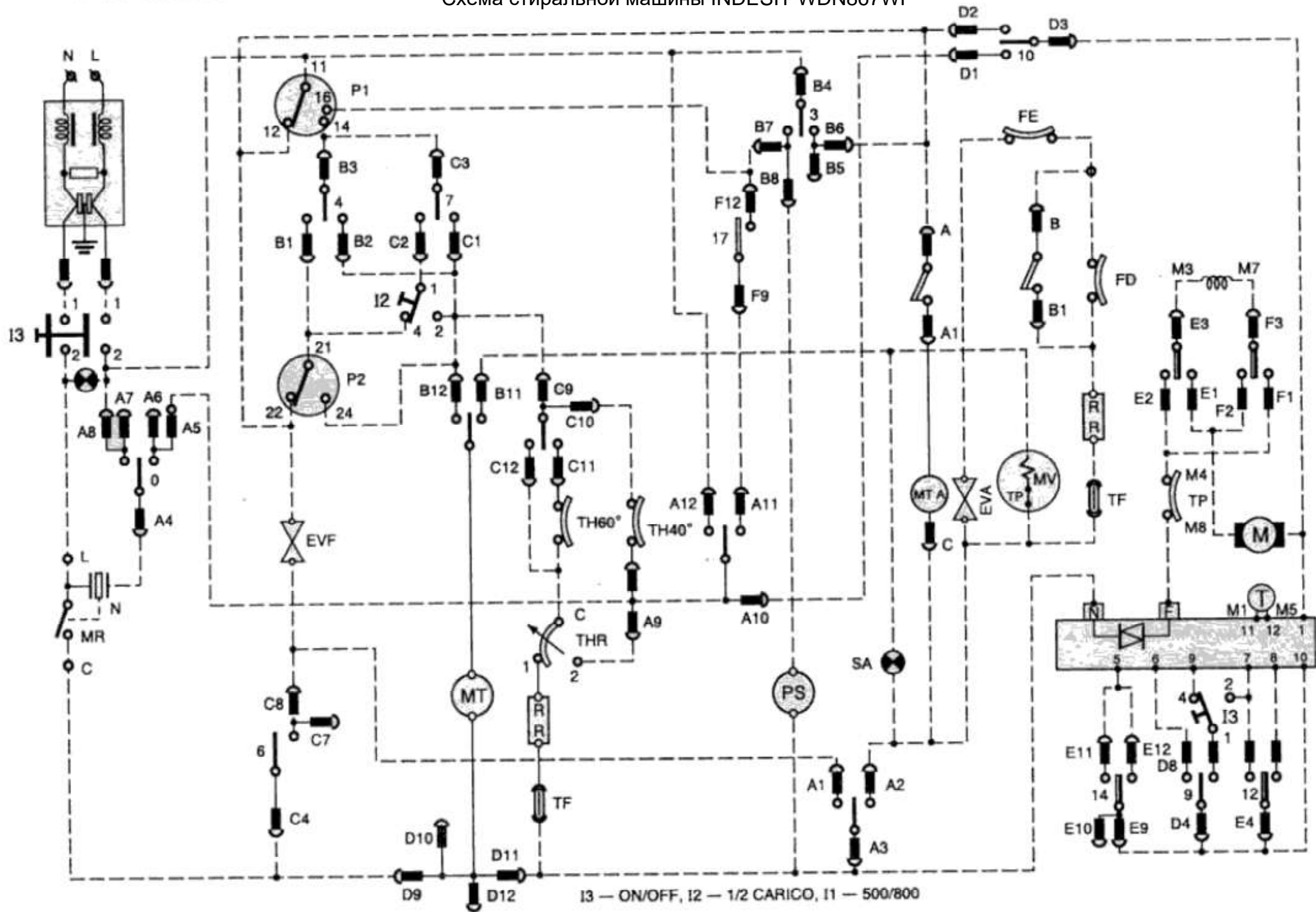
Электрическая схема стиральной машины INDESIT WDN867WF
