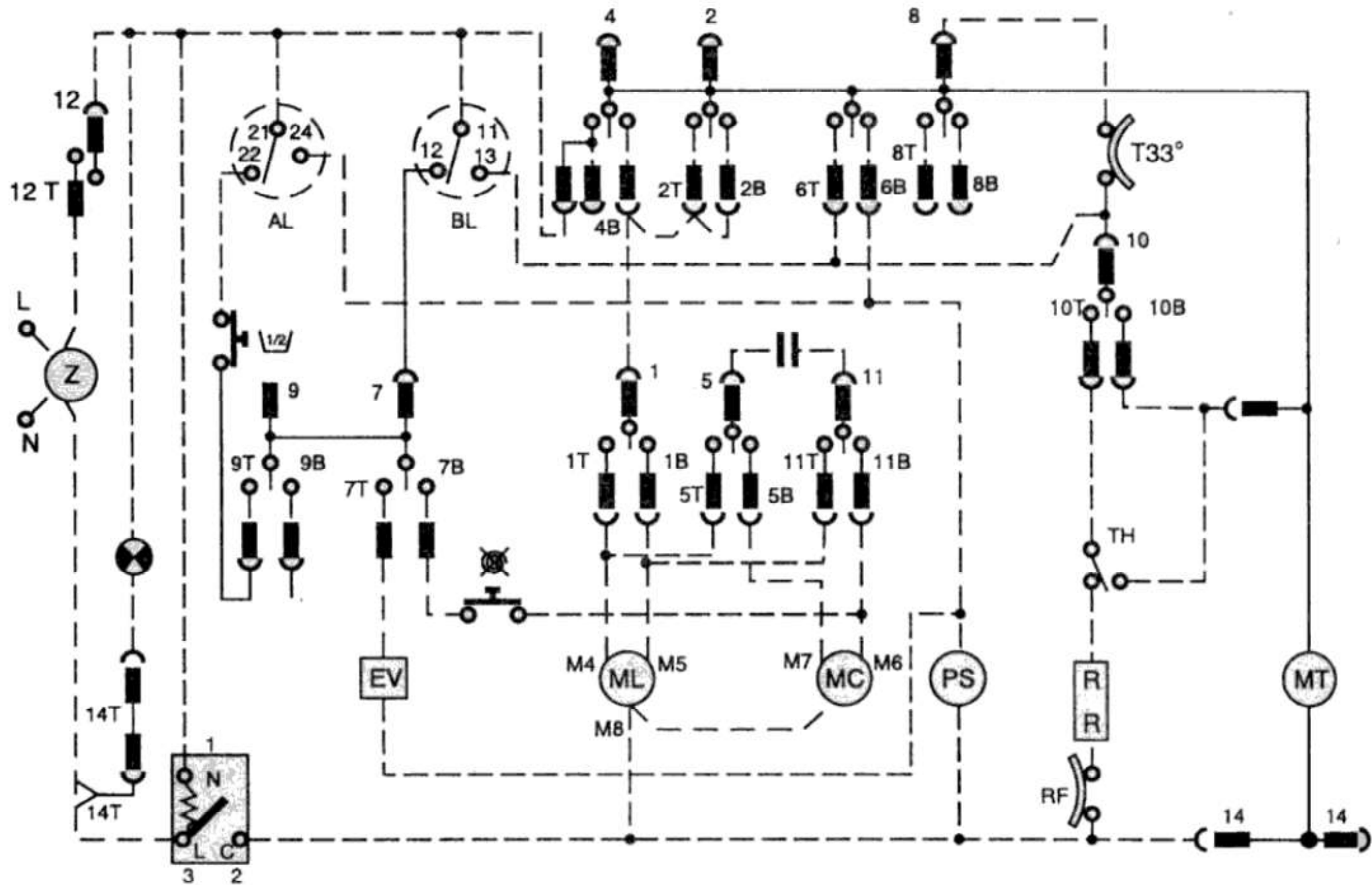
Электрическая схема стиральной машины INDESIT WT600U
