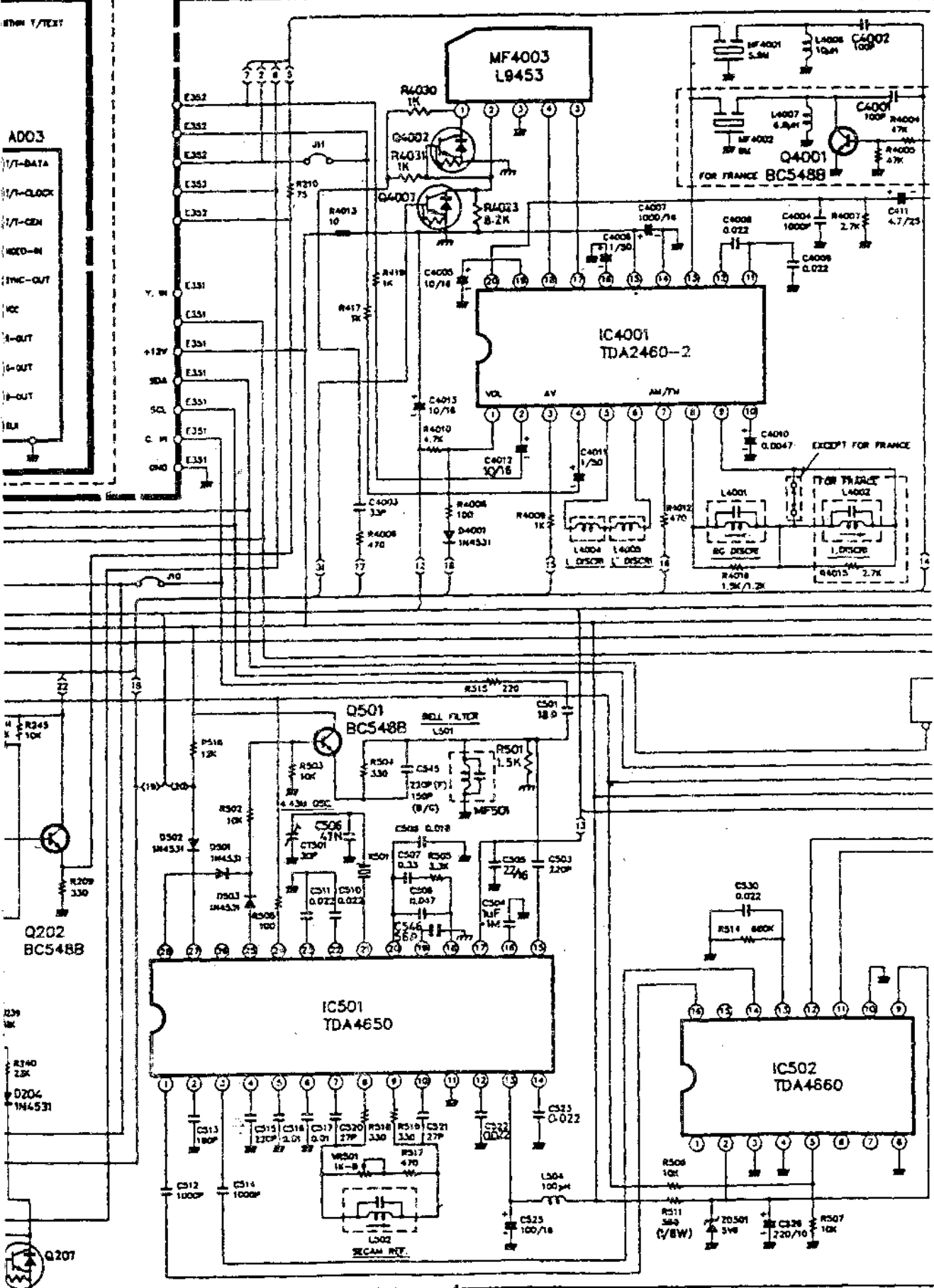
Схема телевизора Hitachi 1408RX, 1408TY
