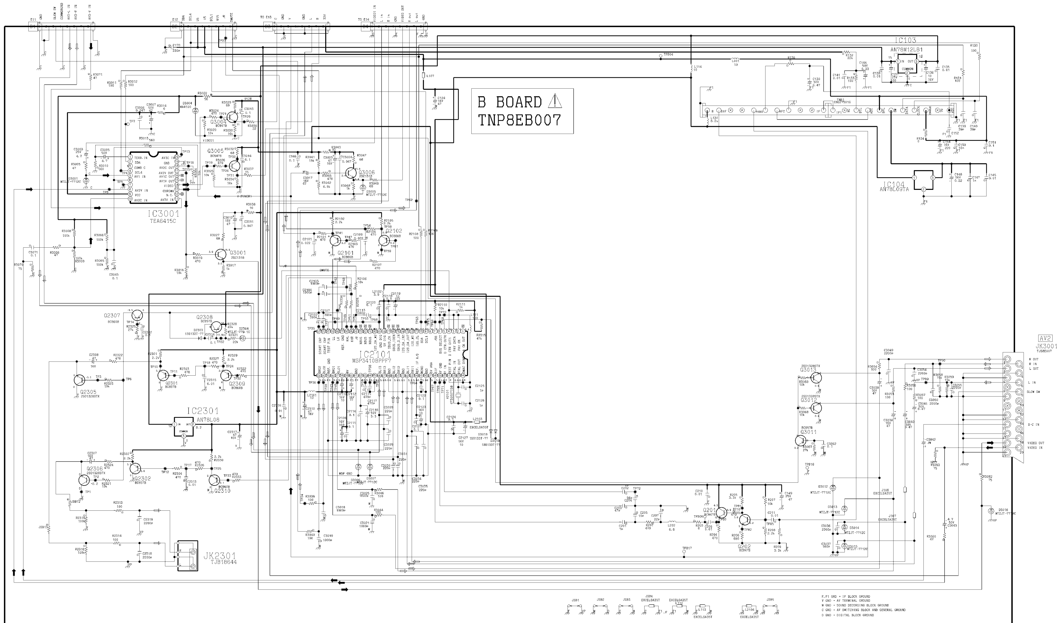
Схема телевизора Panasonic TX-21AD2
