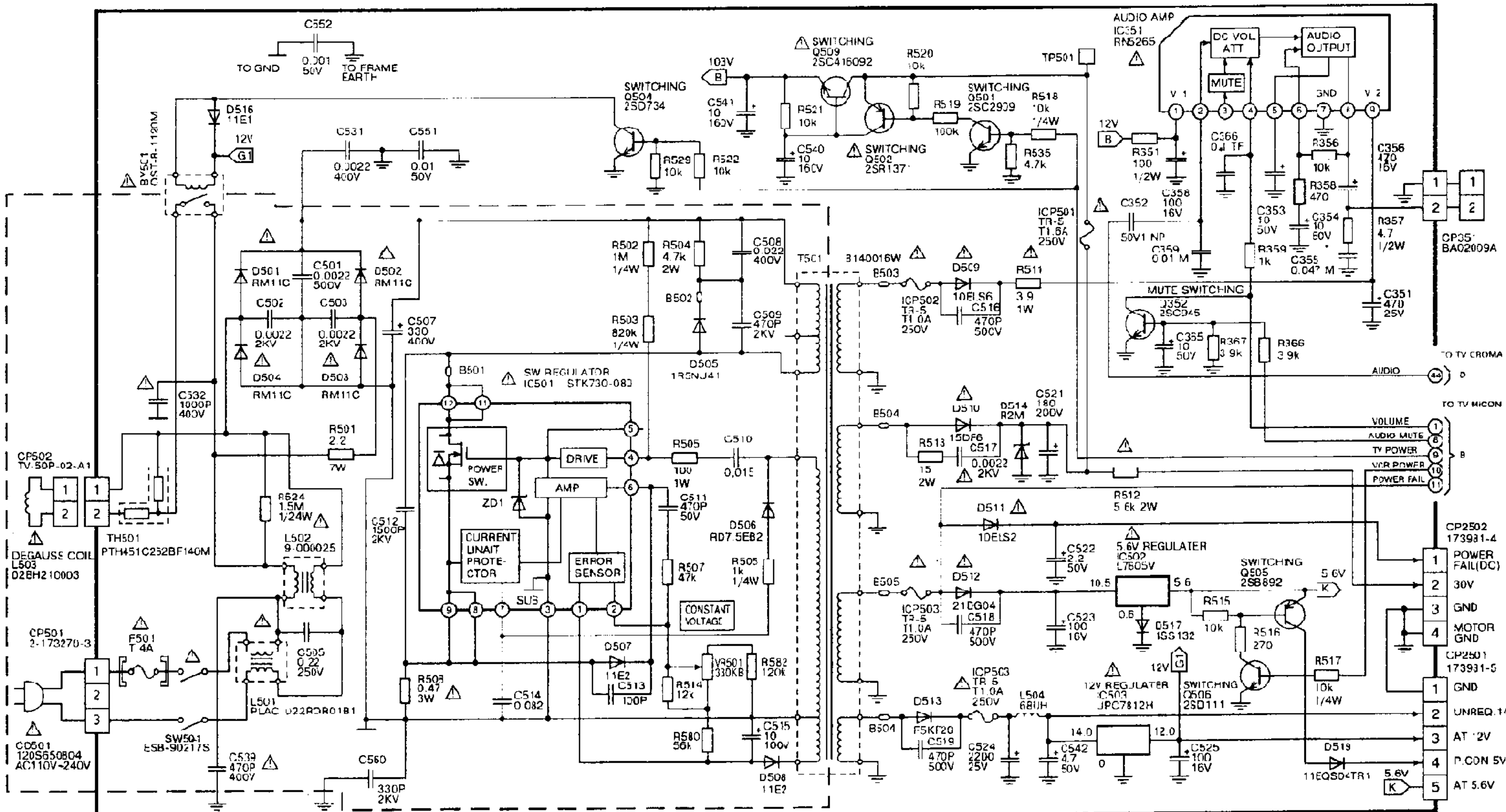
Схема блока питания телевизора AIWA VX-T2020 Электрическая принципиальная схема источника AIWA VX-T2020
