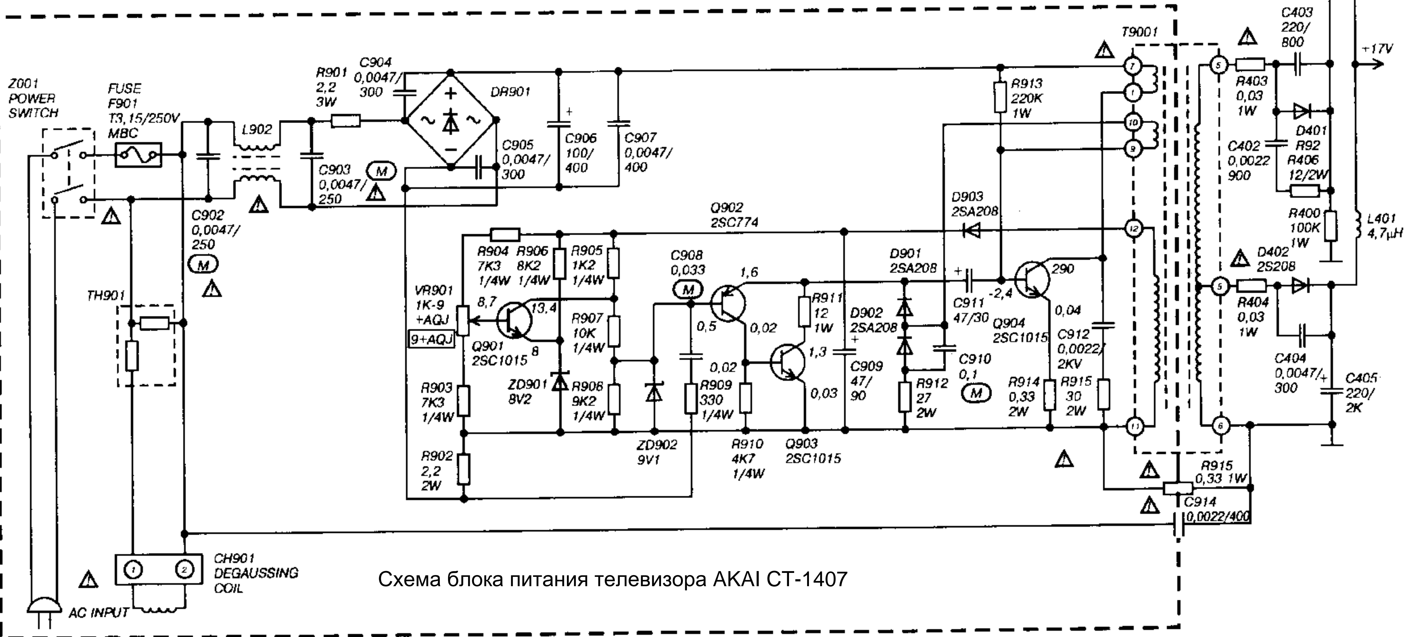
Схема электрическая принципиальная источника питания телевизора AKAI CT-1407
