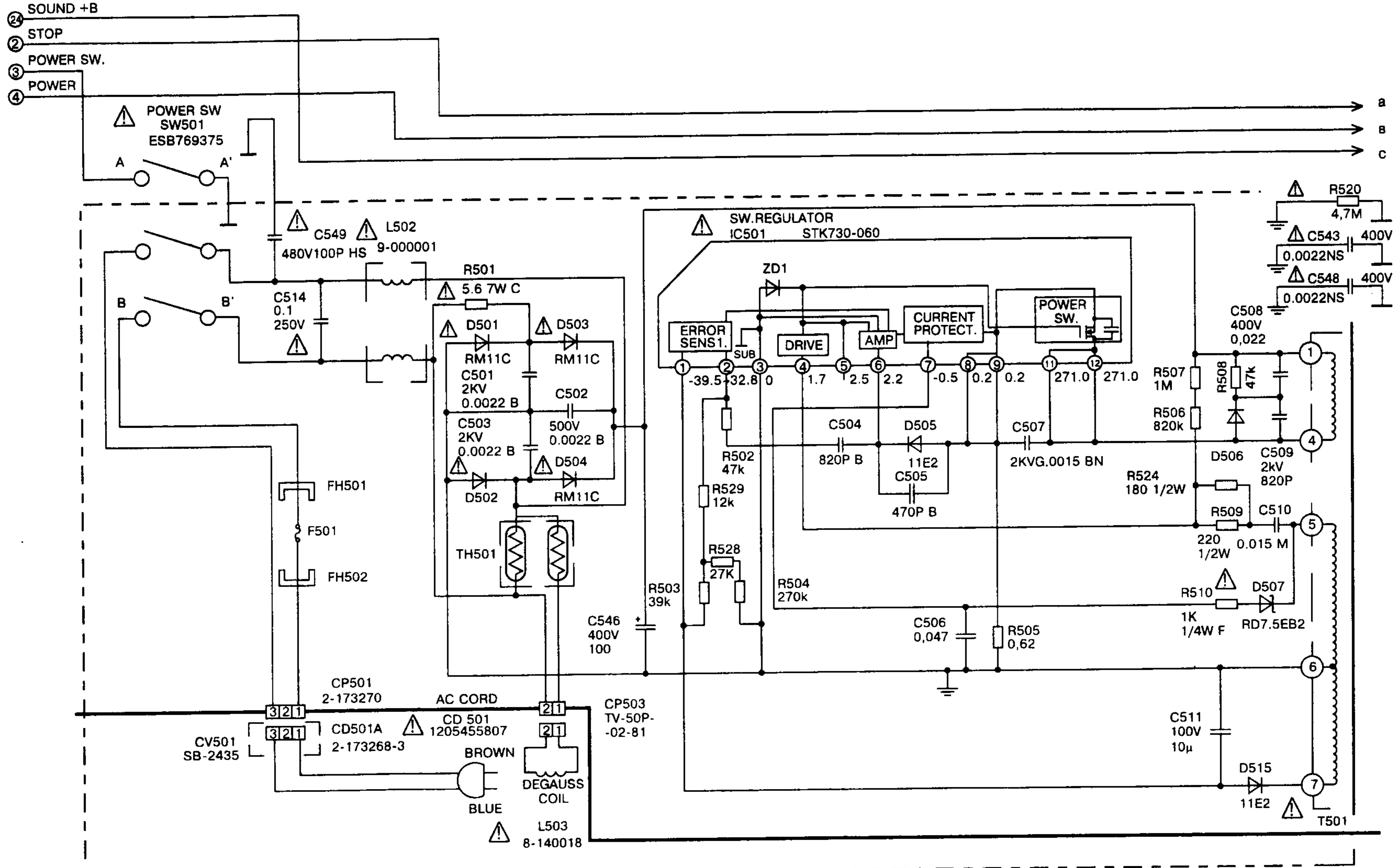
Схема блока питания телевизора АТЕС TV 1402МК9
