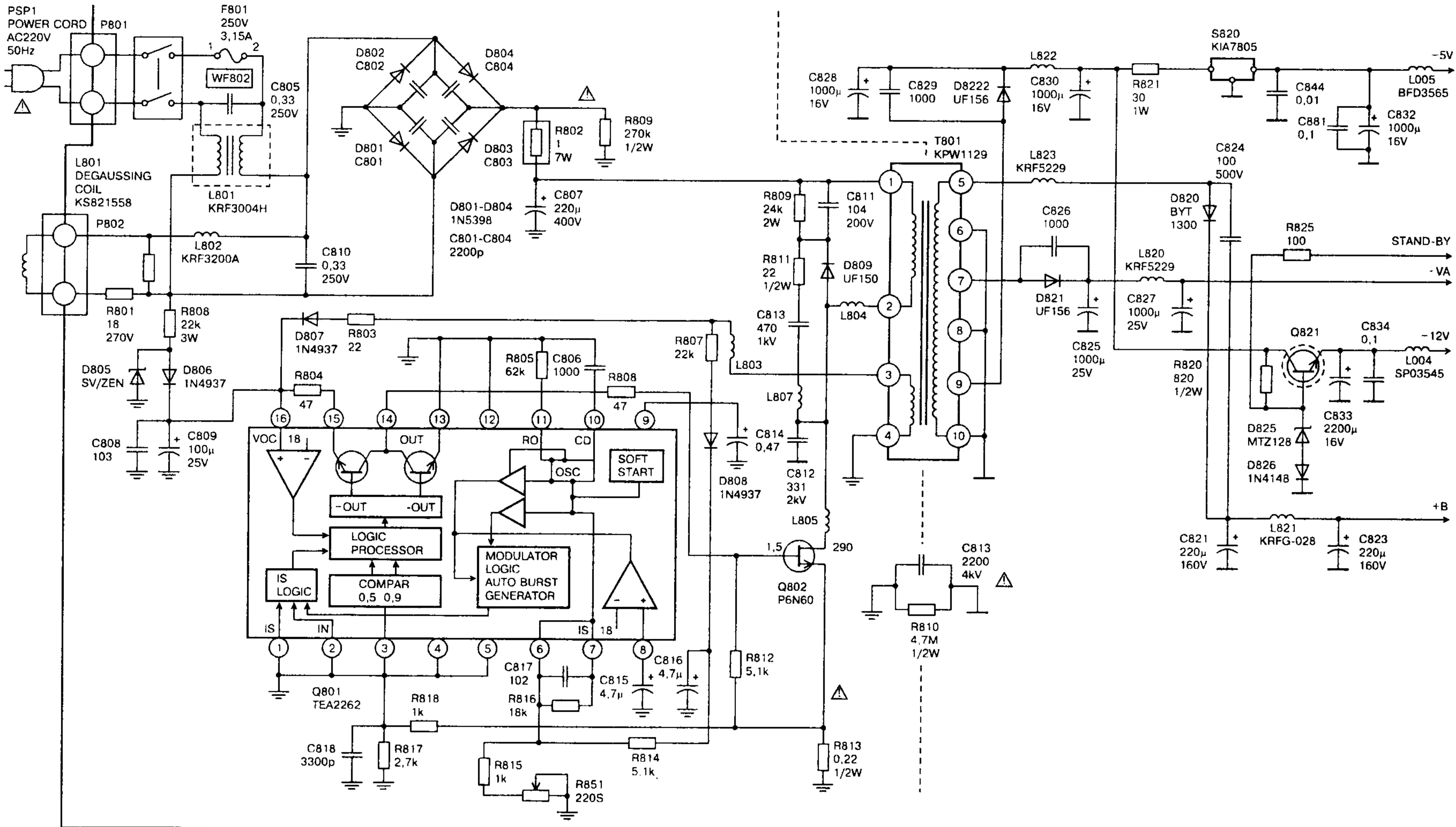
Схема блока питания телевизора ELEKTA CTR-20T
