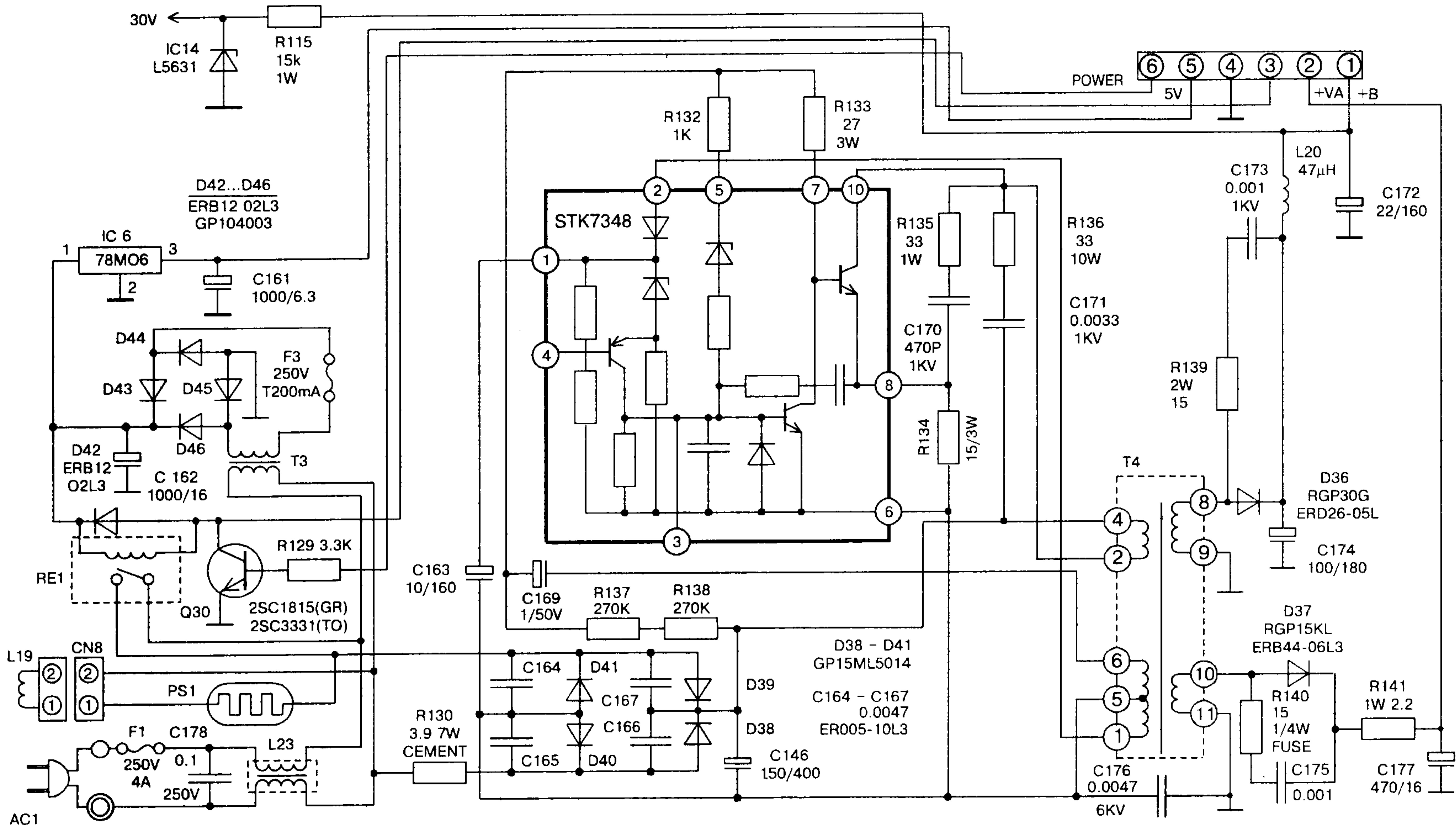
Схема блока питания телевизора FUNAI TV-2003/TV-20MS
