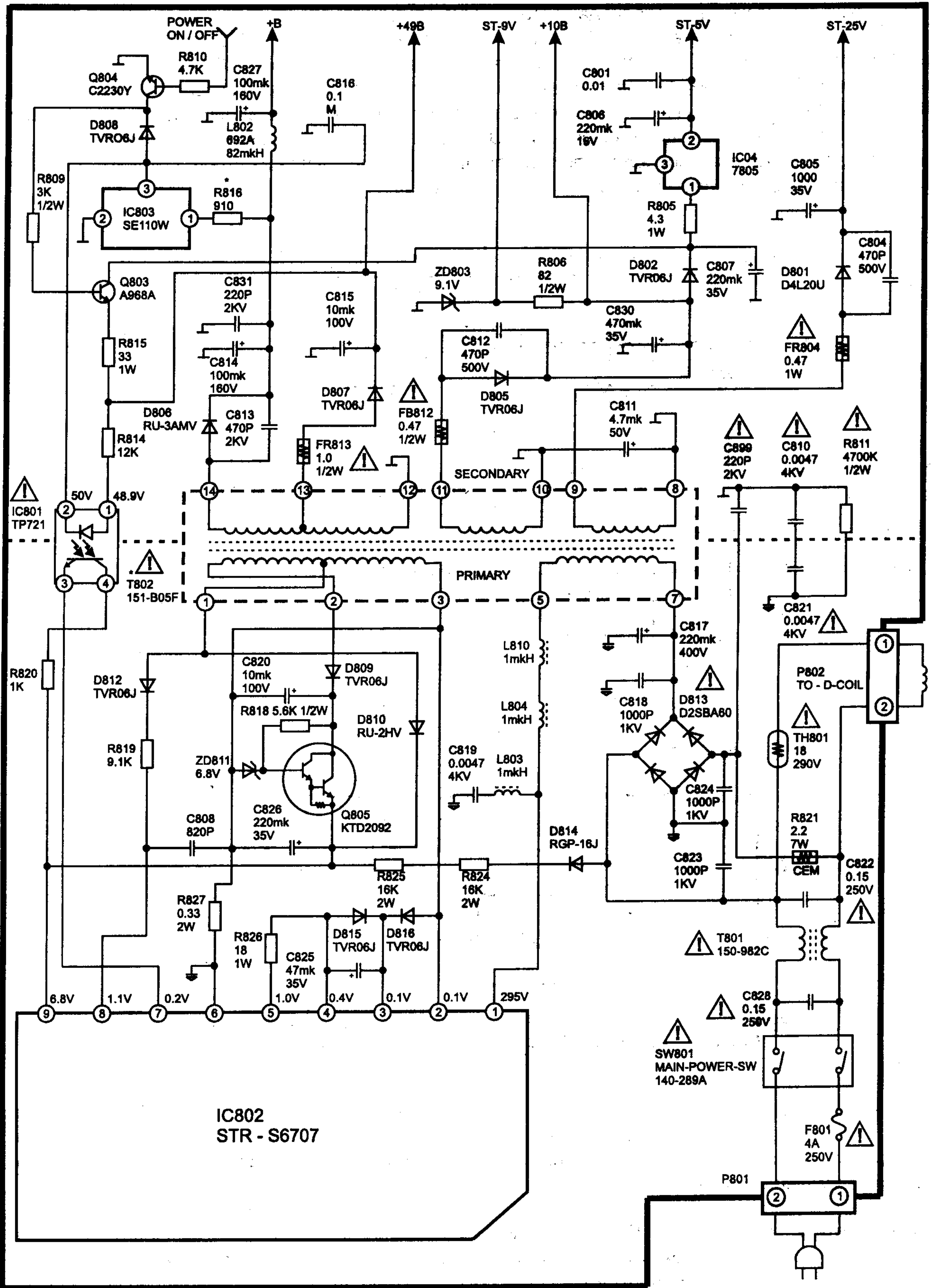
Принципиальная схема
