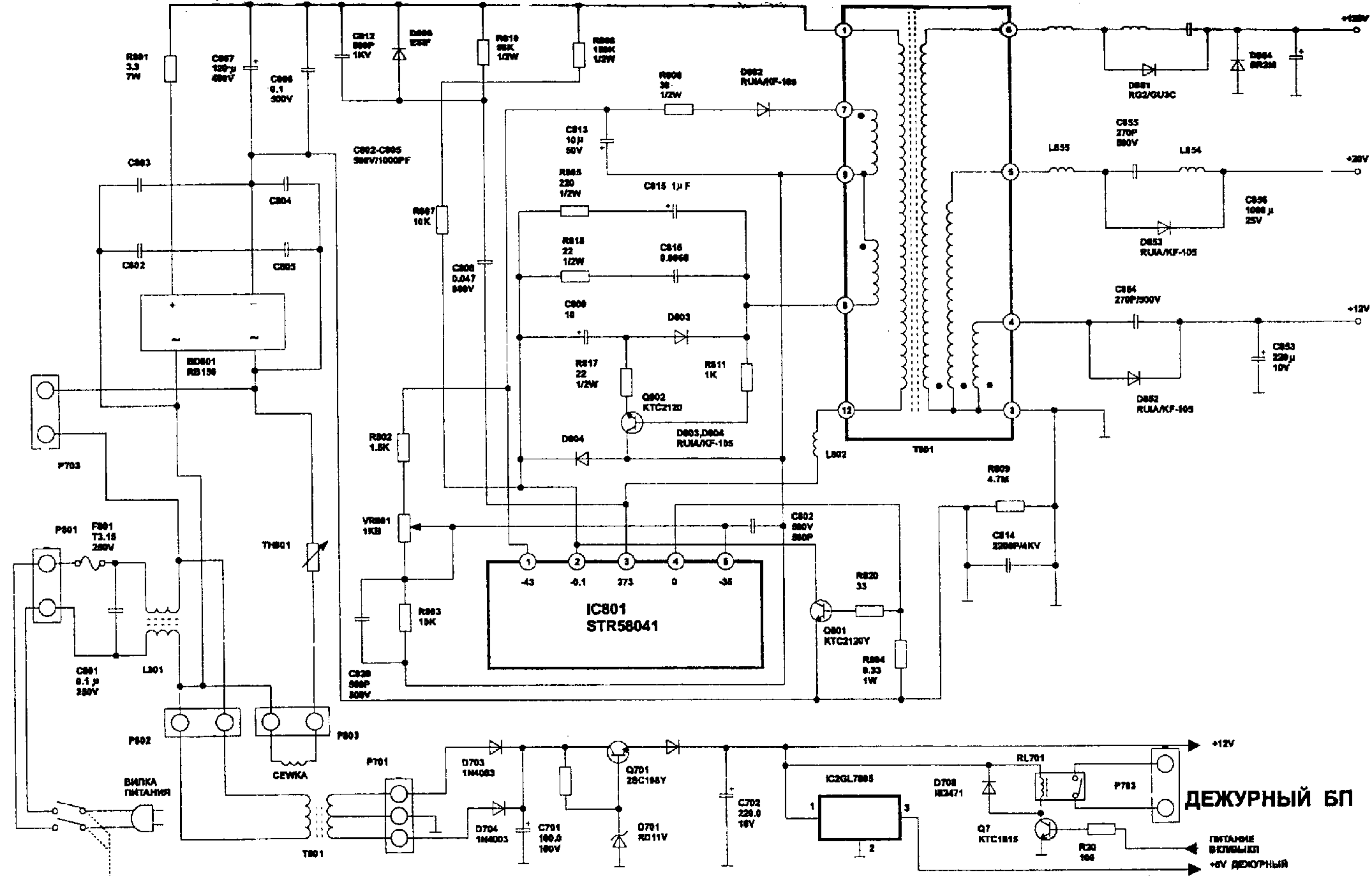
Схема блока питания телевизора GOLDSTAR CF-14A80V
