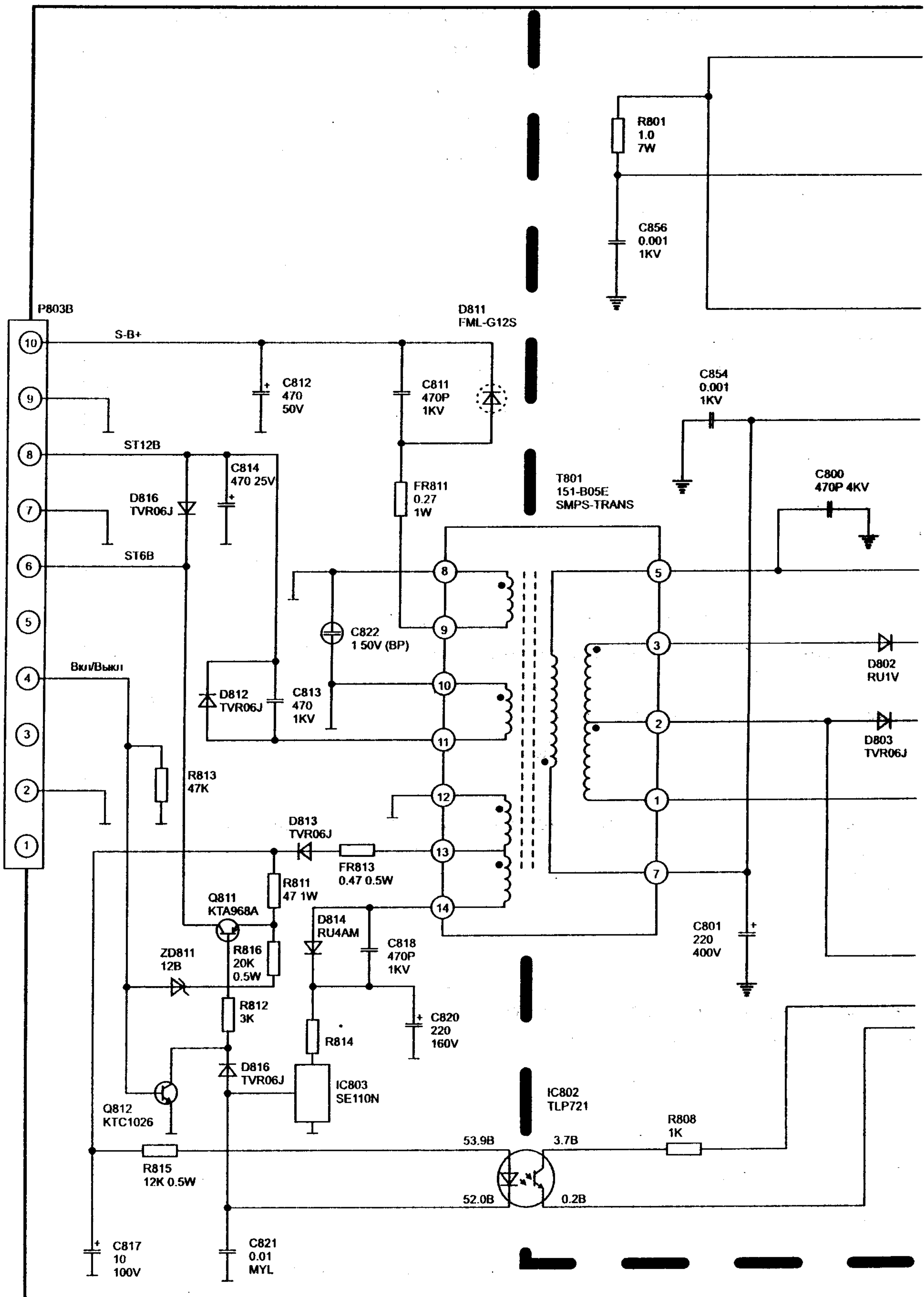
Принципиальная схема
