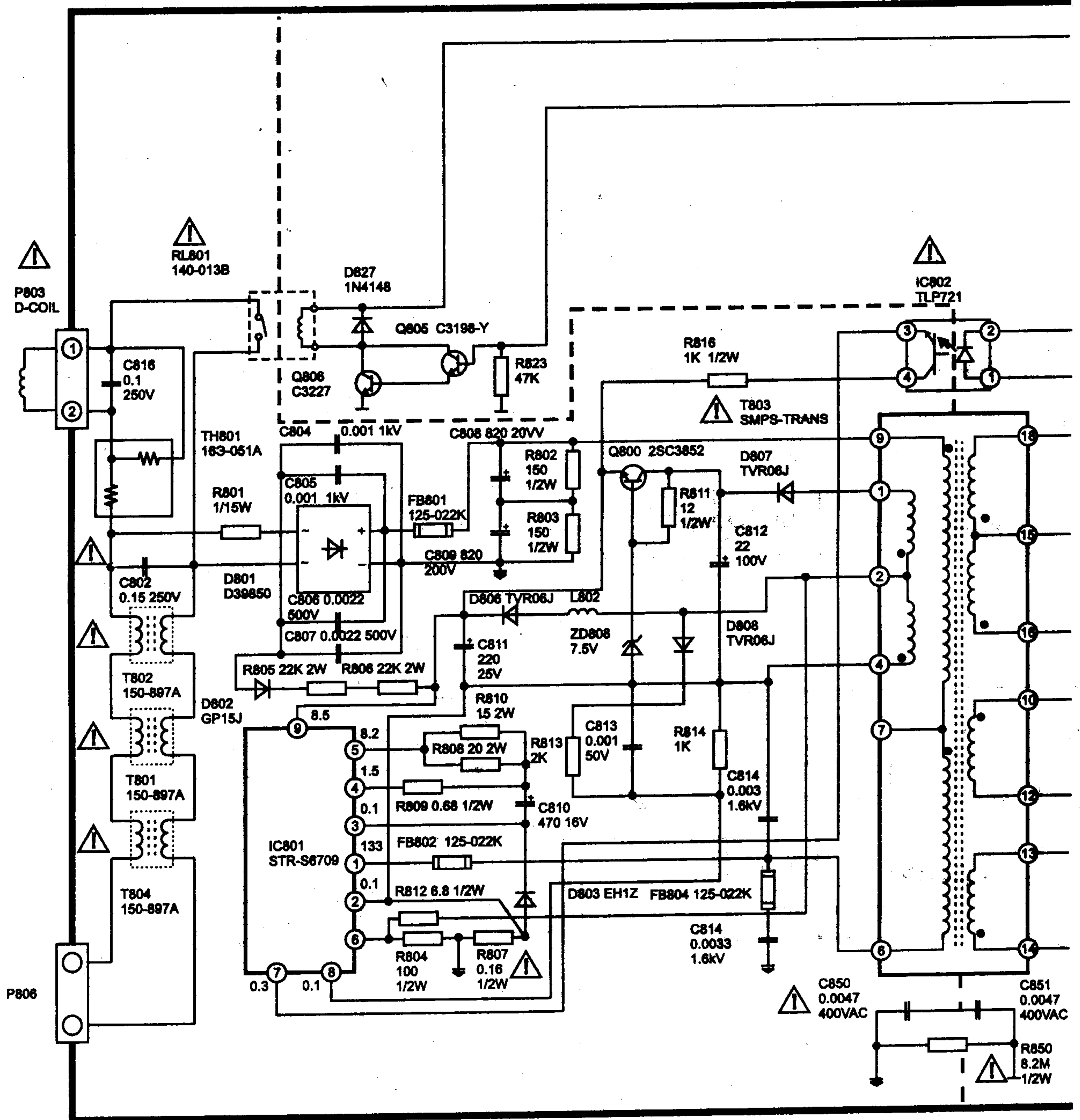
Принципиальная схема
