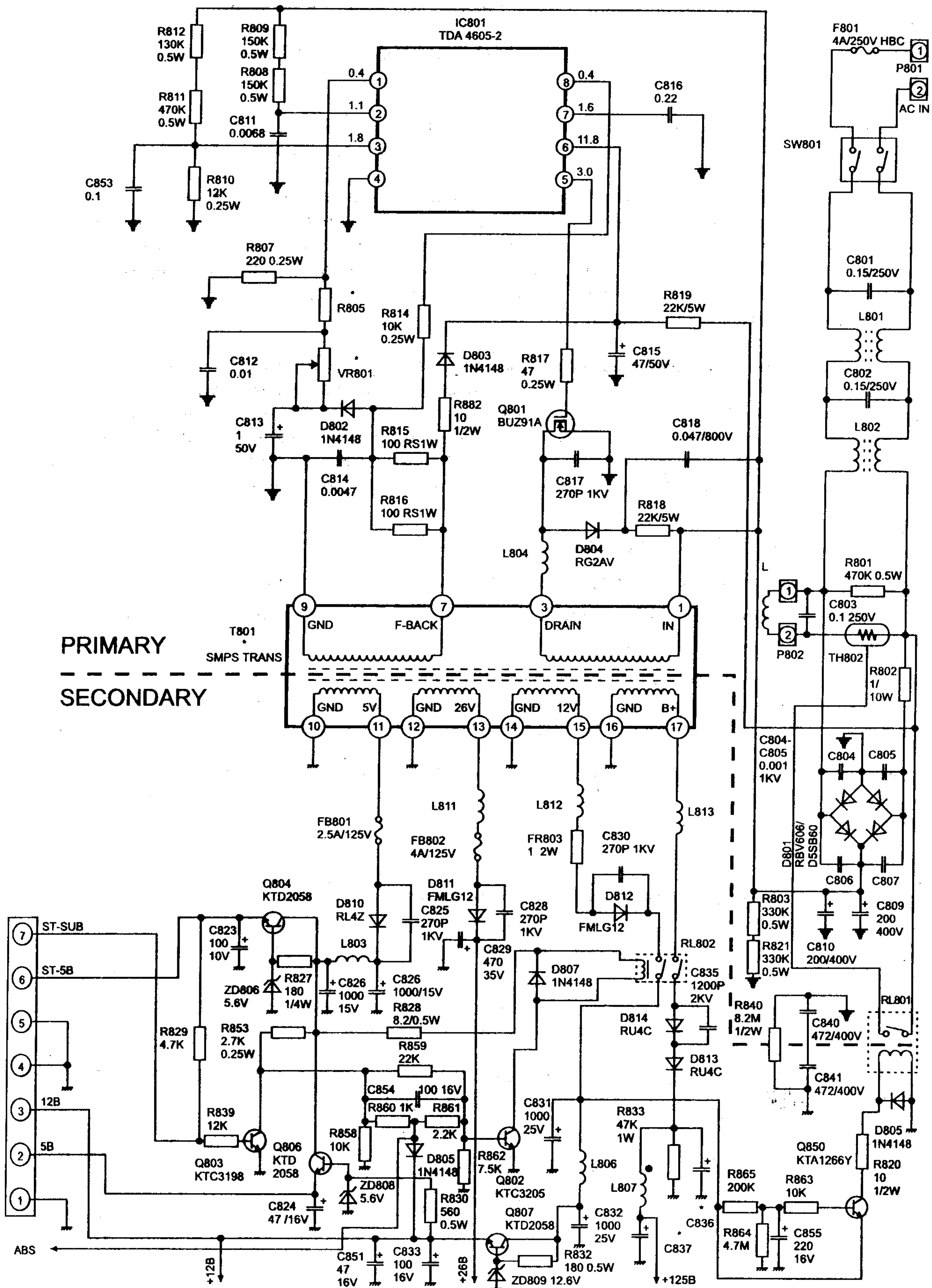
Принципиальная схема
