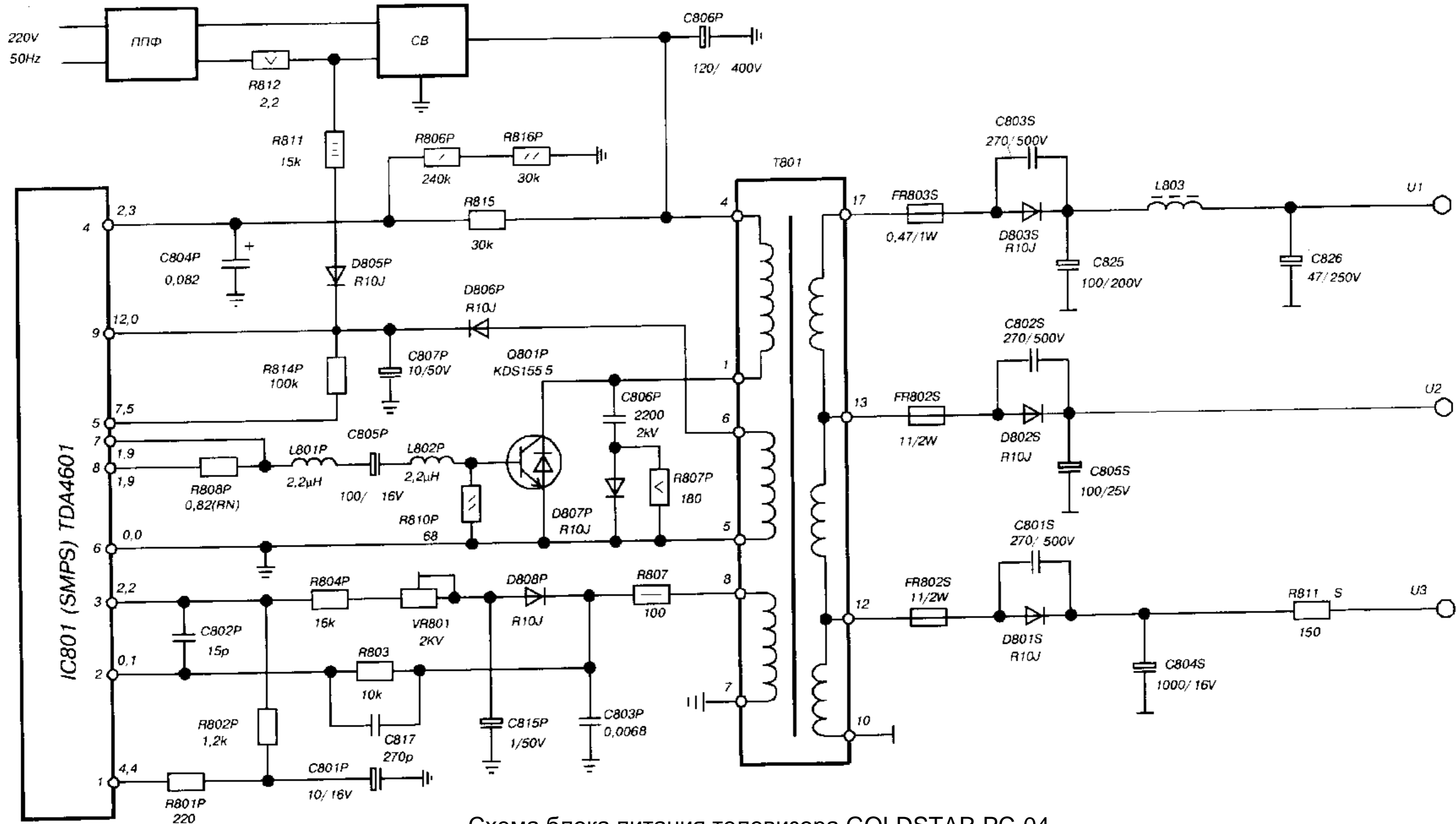
Схема блока питания телевизора GOLDSTAR PC-04 Импульсный источник питания телевизора "GOLDSTAR PC-04"
