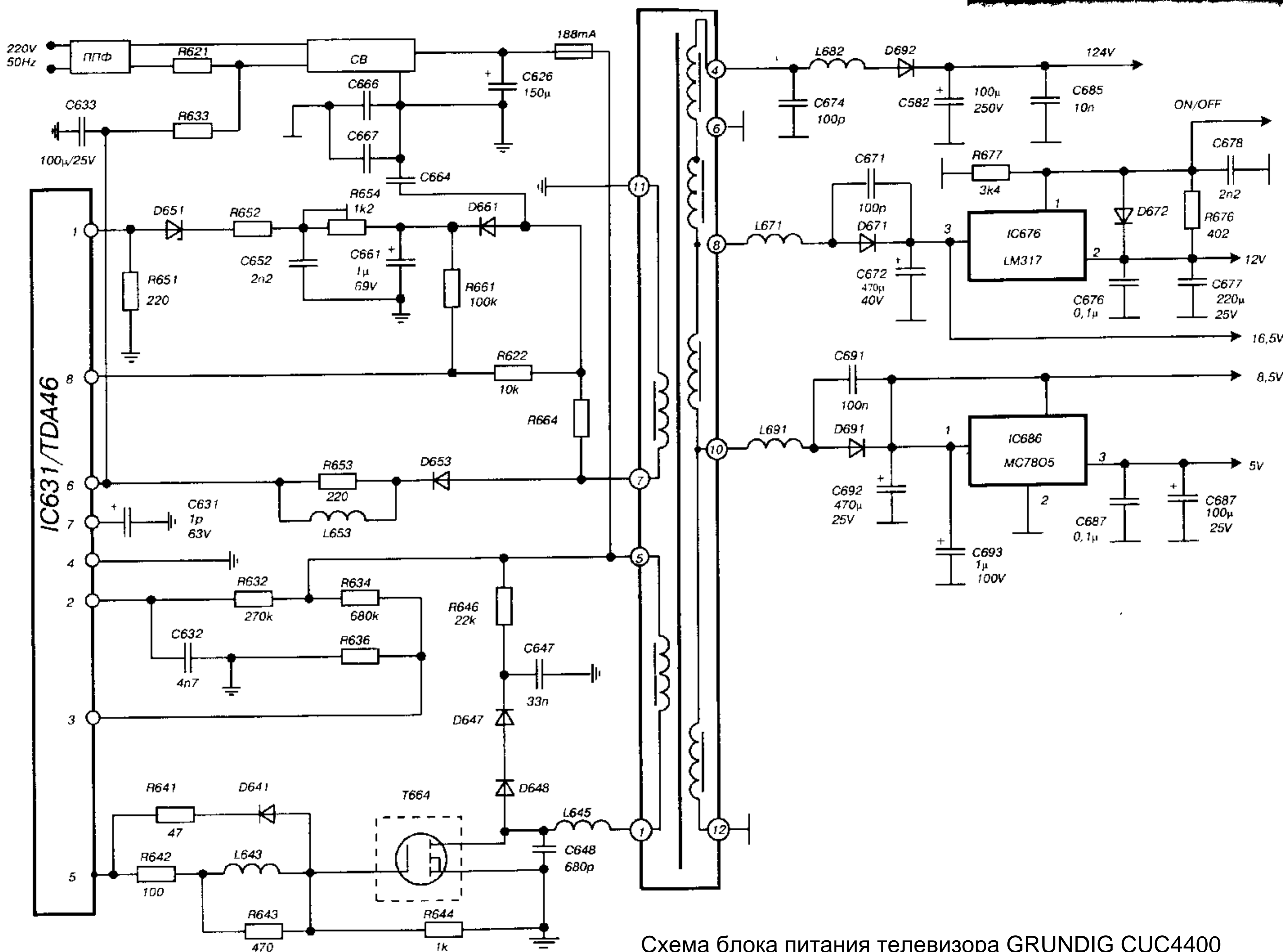
Импульсный источник питания телевизора "GRUNDIG CUC-4400"
