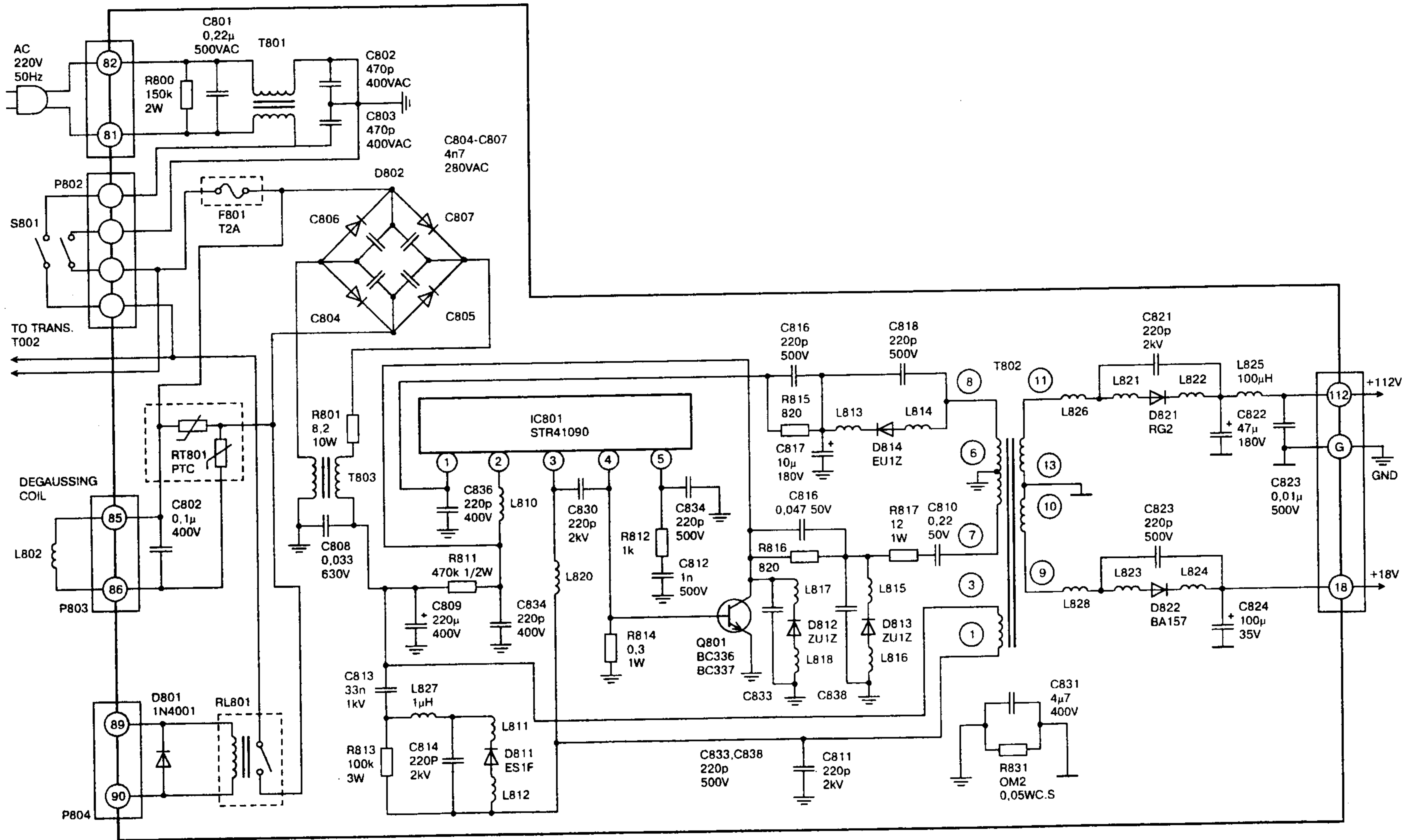
Схема блока питания телевизора НАРПИ
