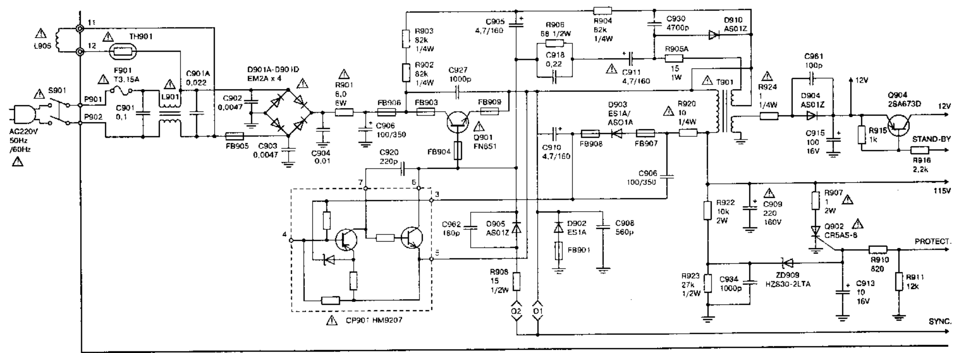
Схема блока питания телевизора HITACHI CMT-2141, CMT-1450
