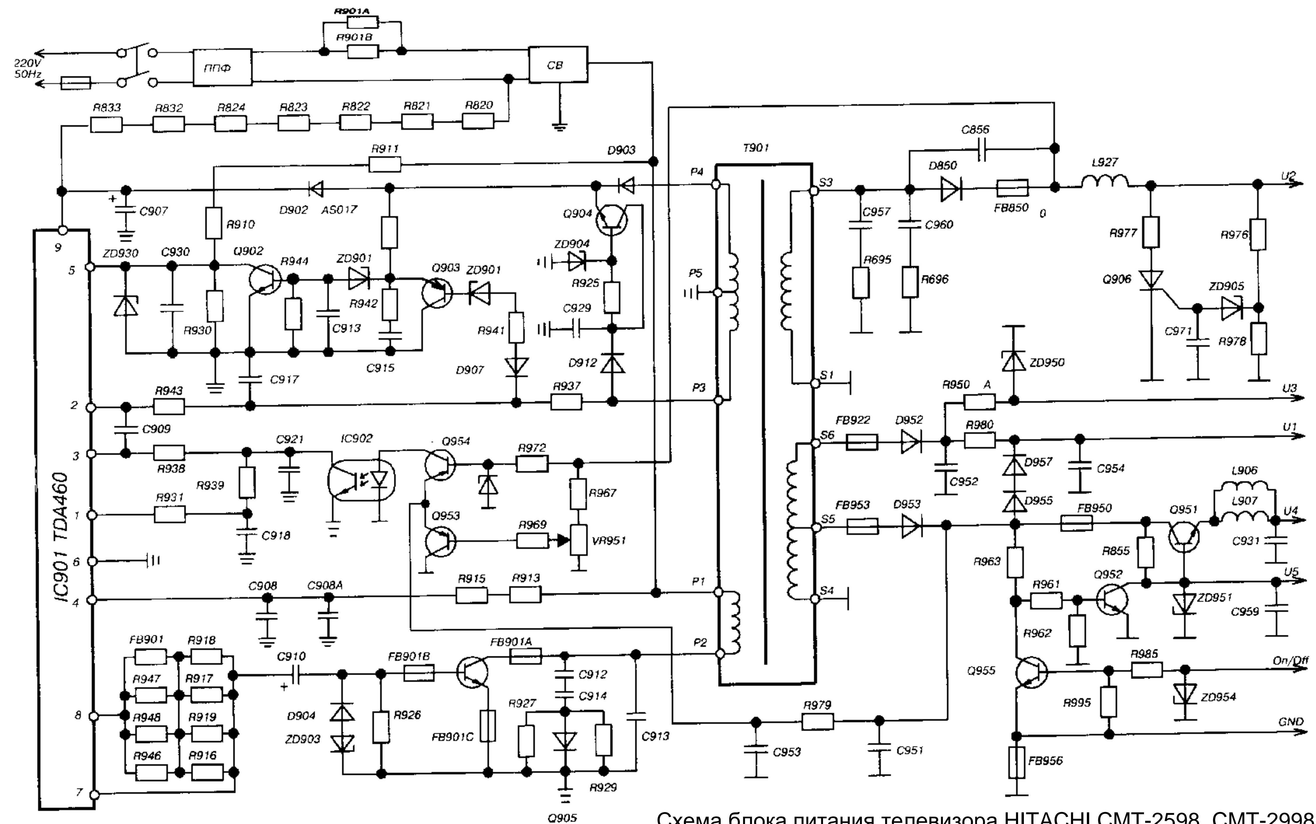
Импульсный источник питания телевизора "HITACHI CMT-2598,2998".
