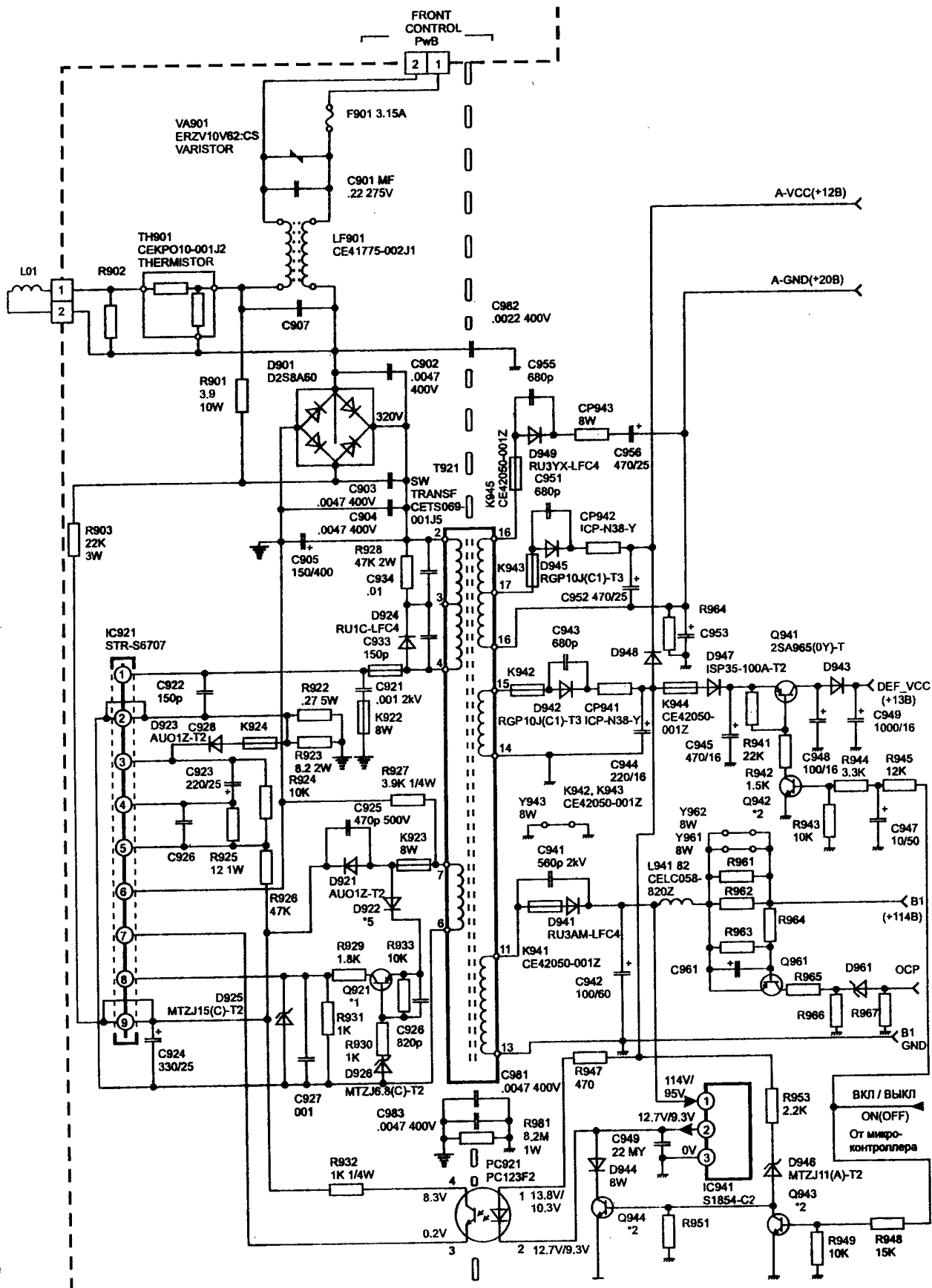
Принципиальная схема
