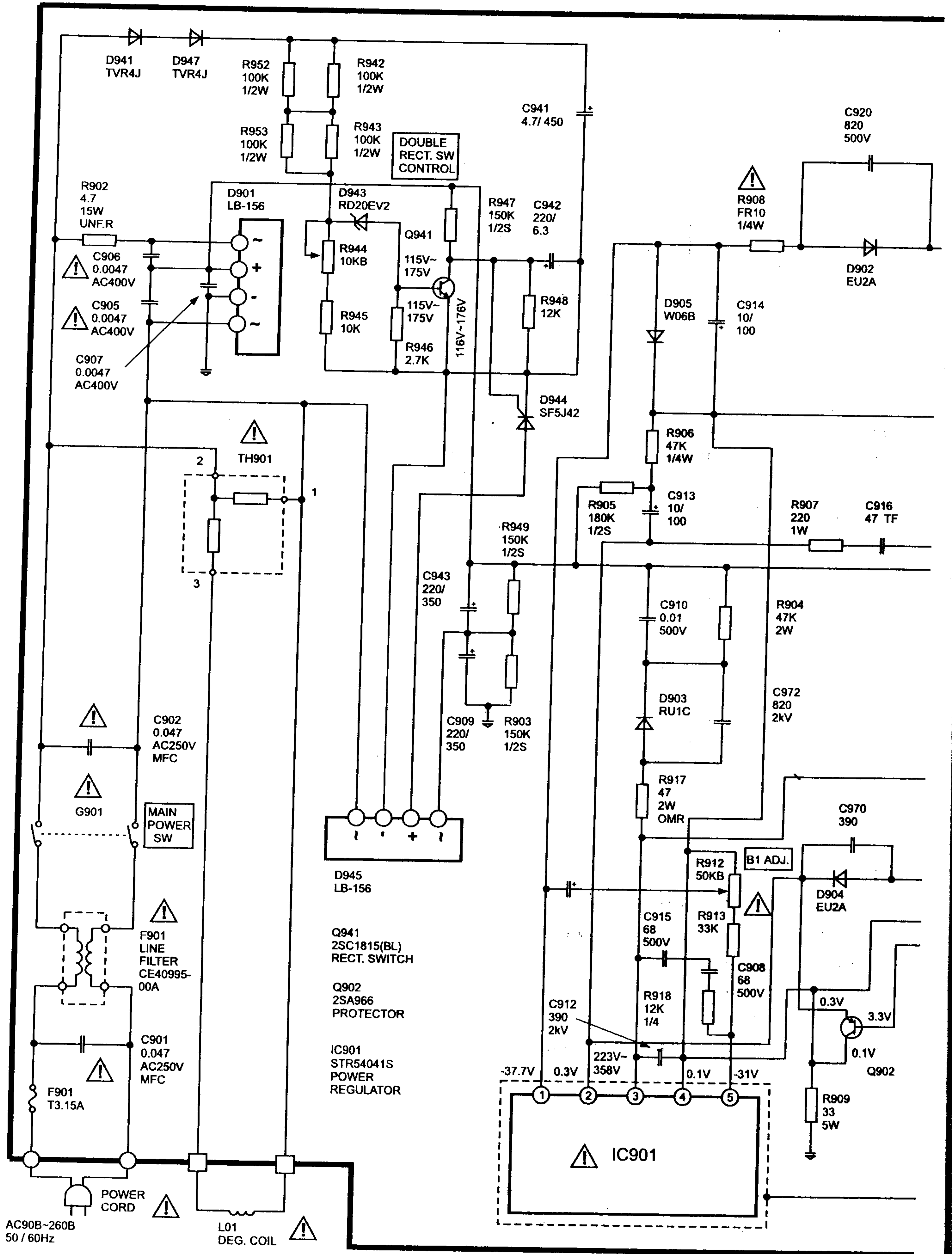
Принципиальная схема
