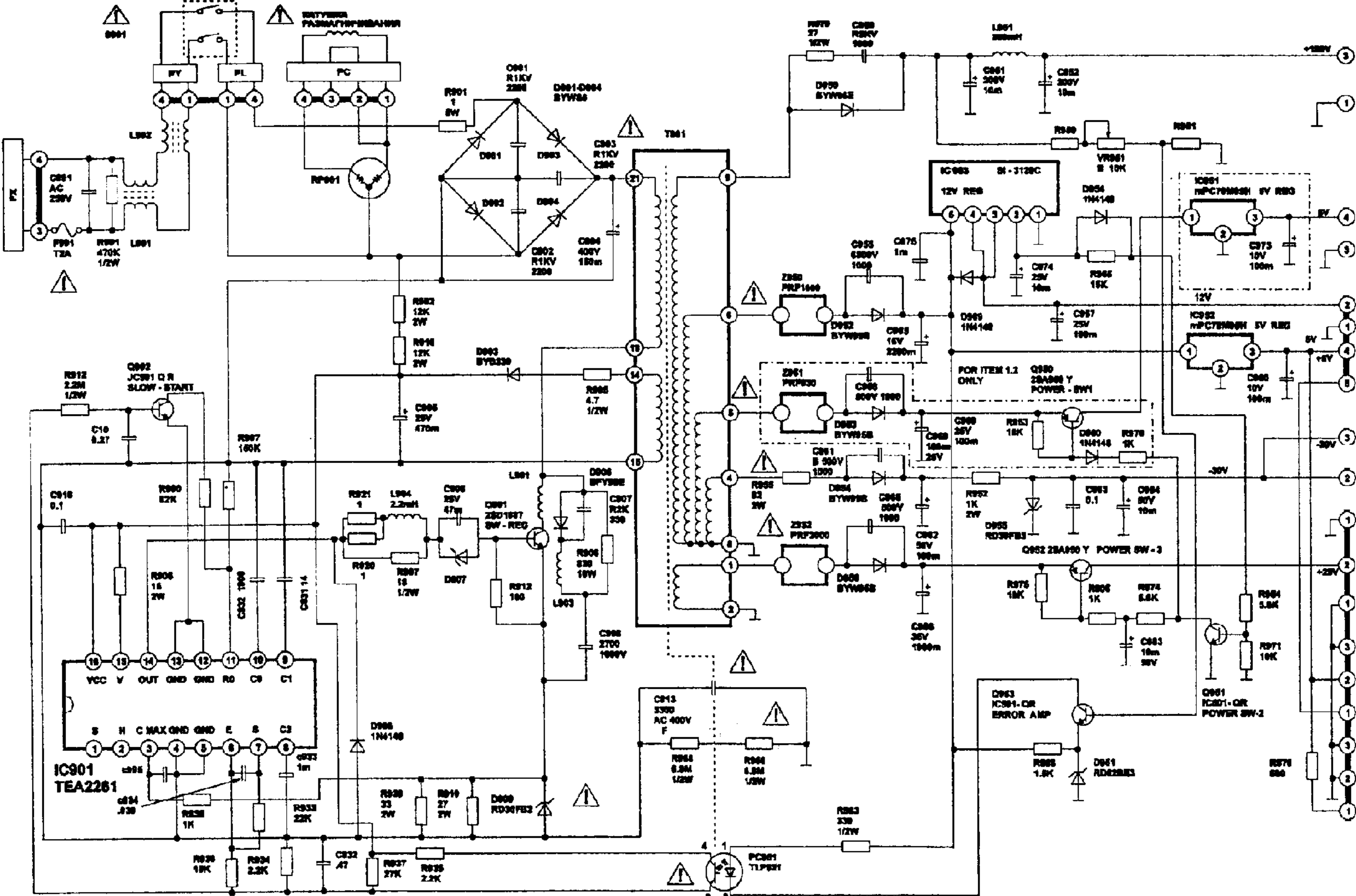
Схема блока питания телевизора MITSUBISHI CT-2125EET
