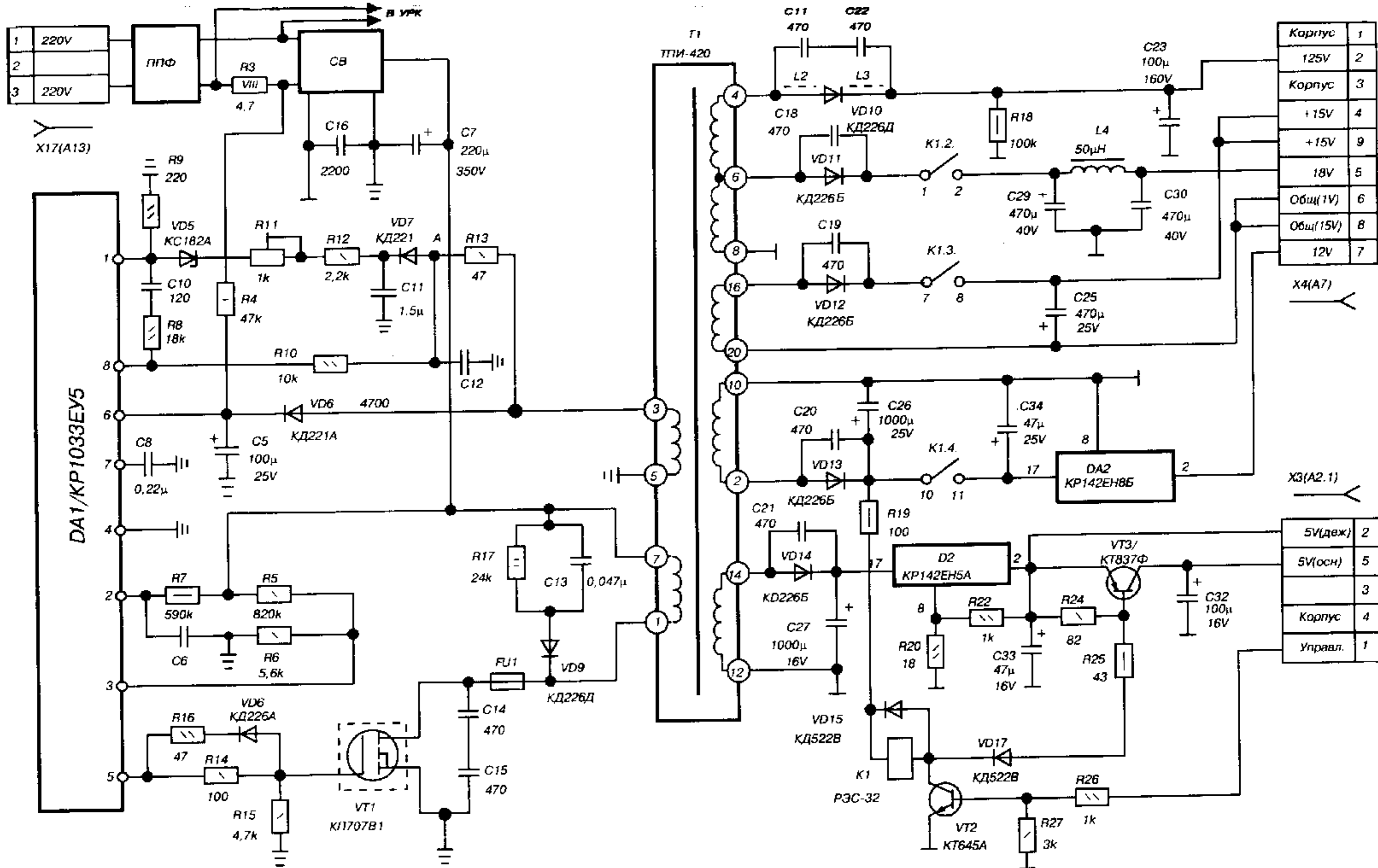
Схема блока питания телевизора МП-420-2
