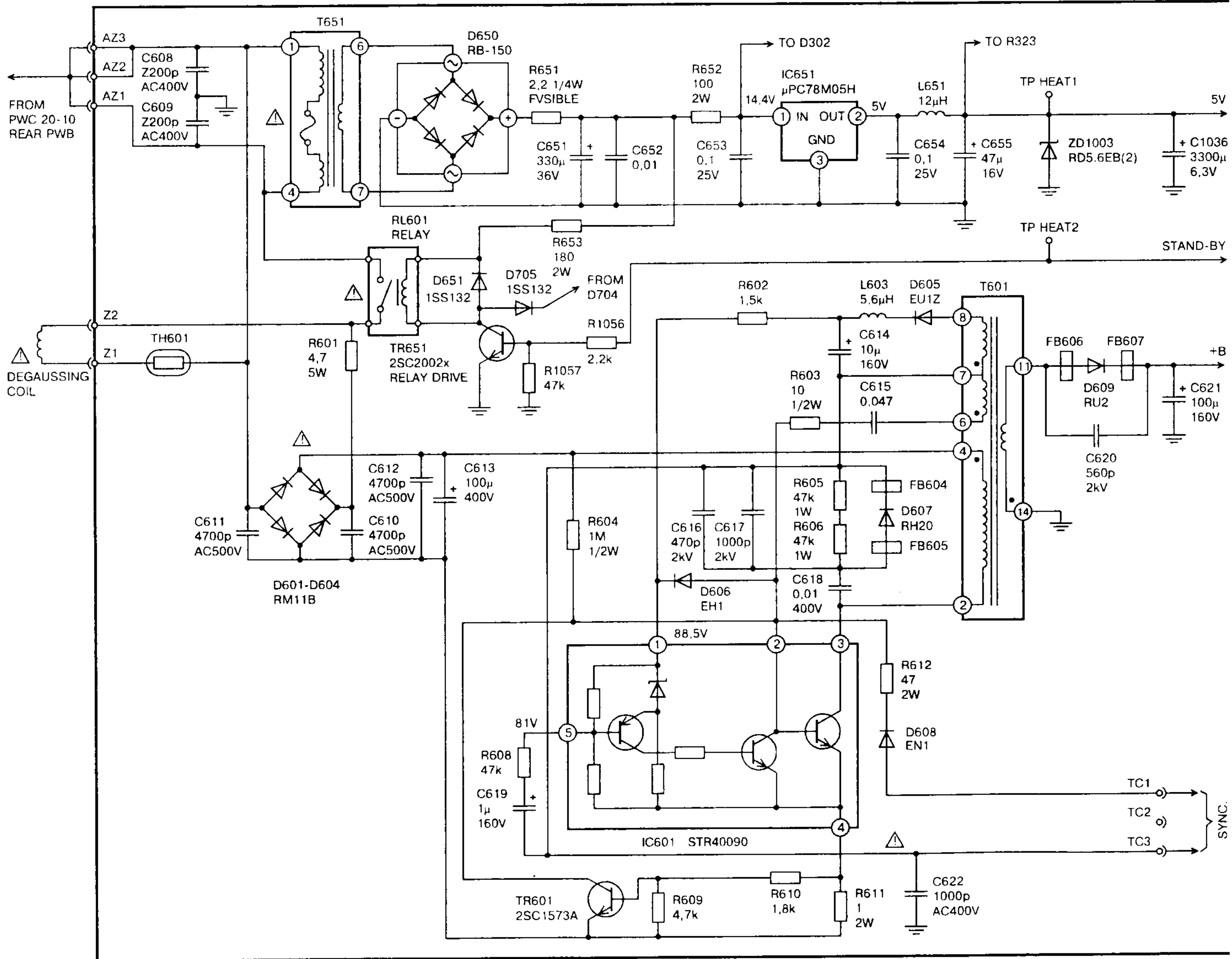
Схема блока питания телевизора NEC FS 1530SK/1530SU
