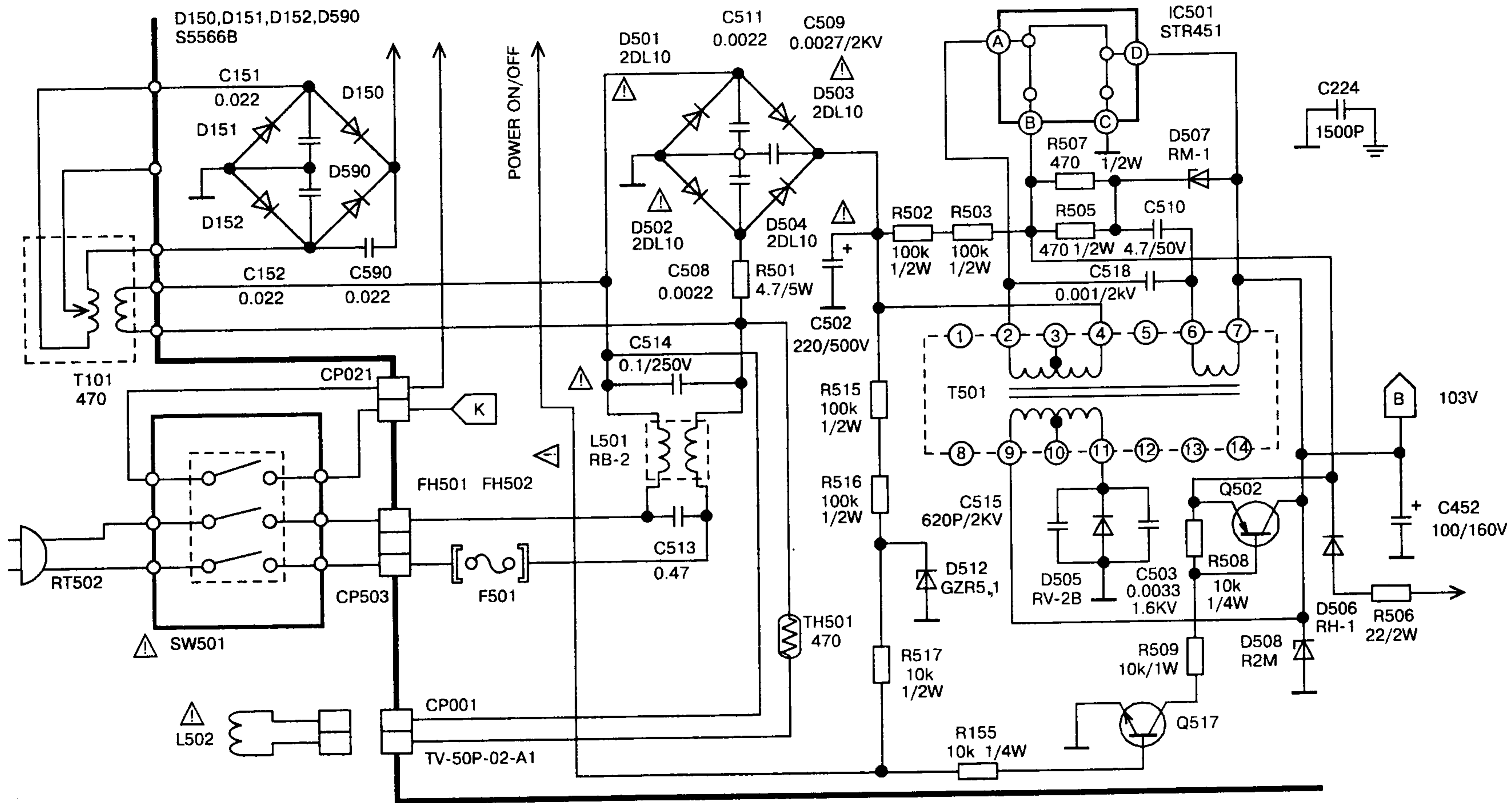
Схема блока питания телевизора ORION 20AH
