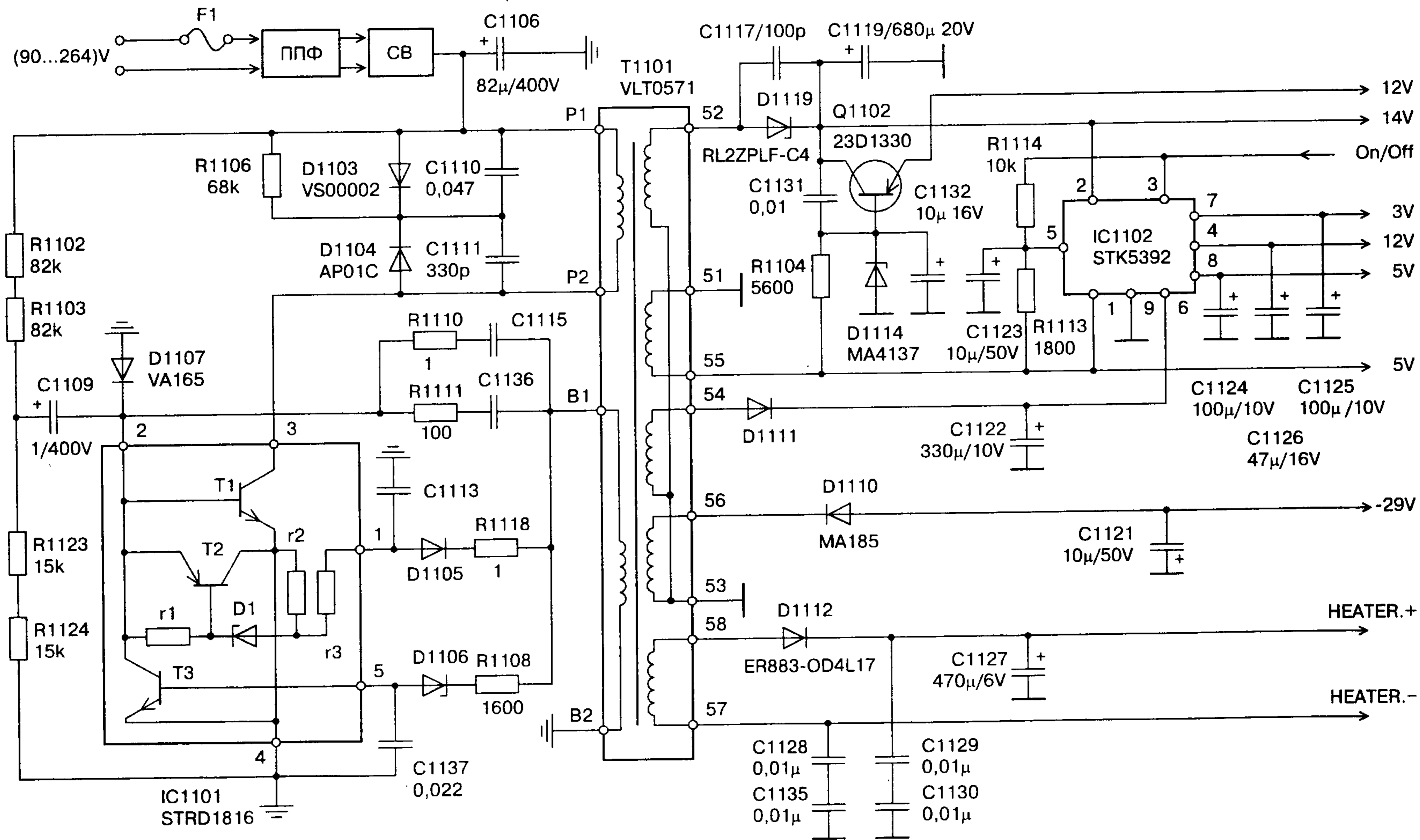
Схема блока питания телевизора PANASONIC NV-J35
